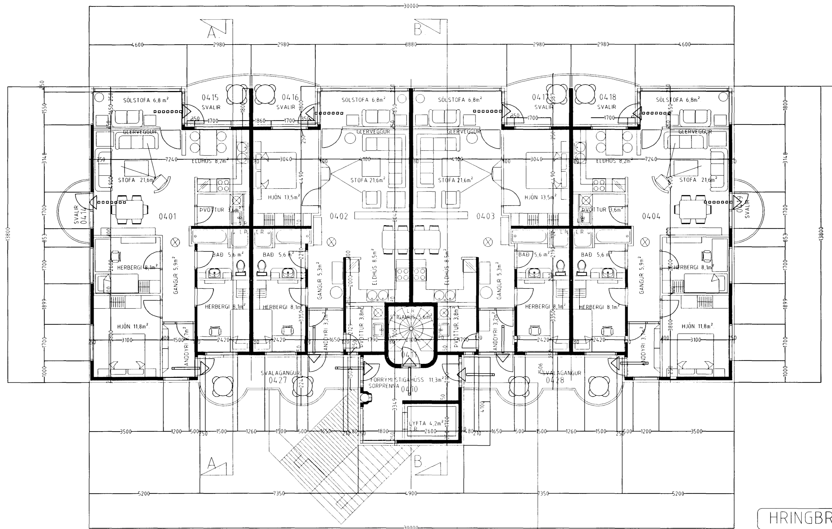
GRUNNMYND 4. HÆÐ m.k.v. 1:100
