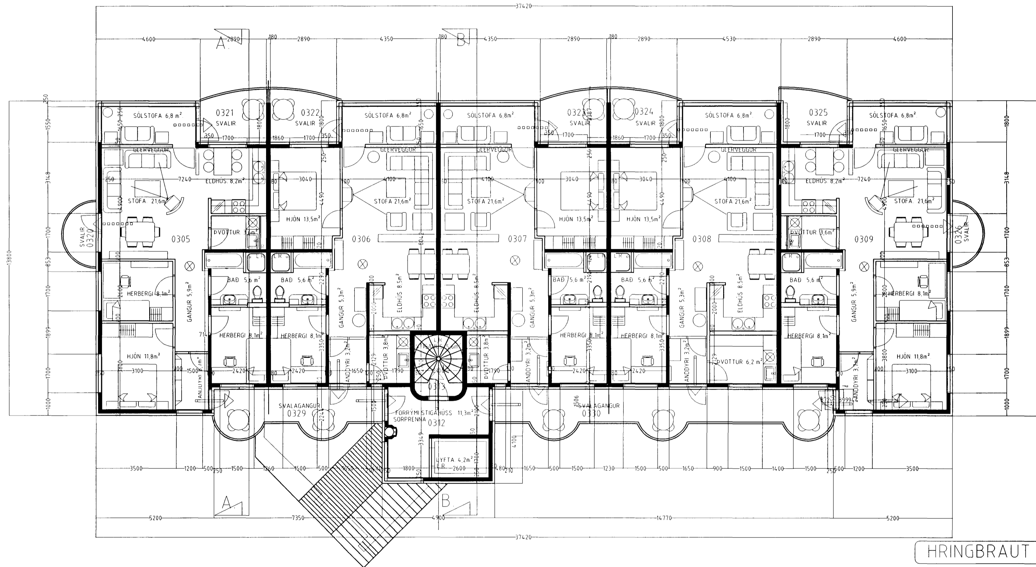
GRUNNMYND 3. HÆÐ. m.kv. 1:100.
