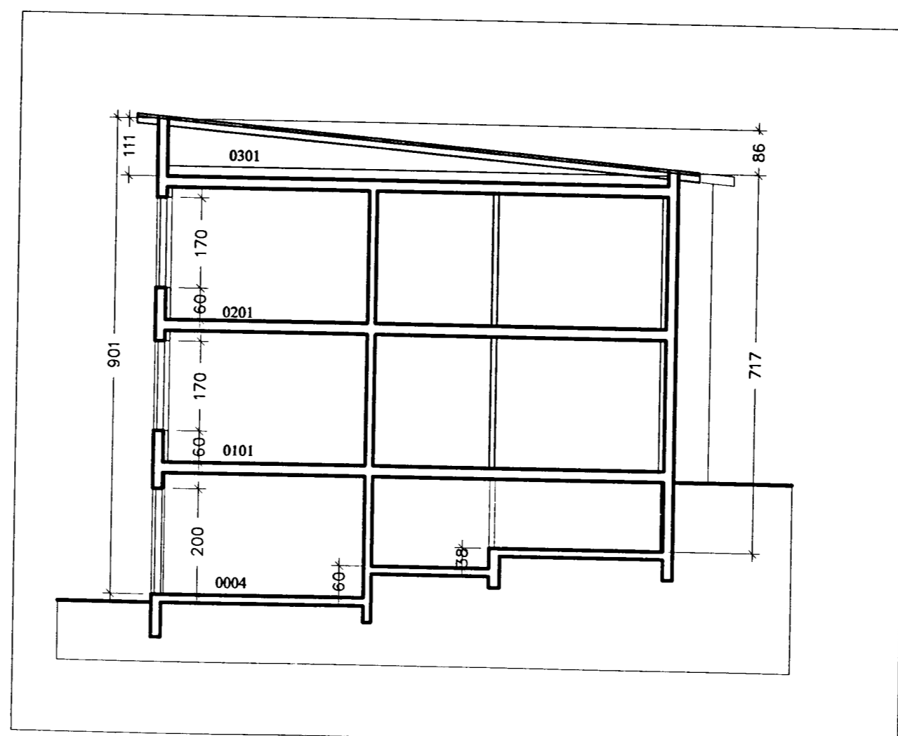
Sneiðing b-b 1:100
