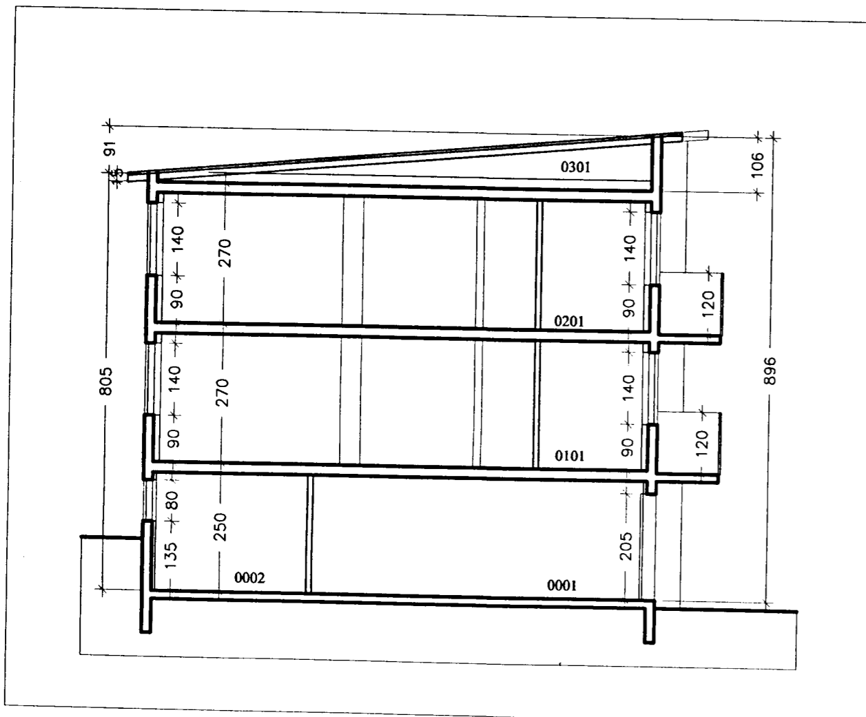
Sneiðing a-a 1:100
