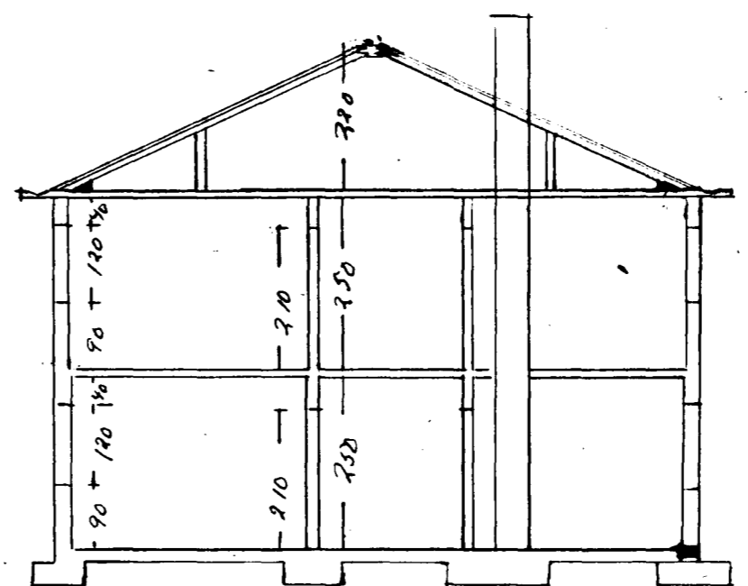
Þverskurður
