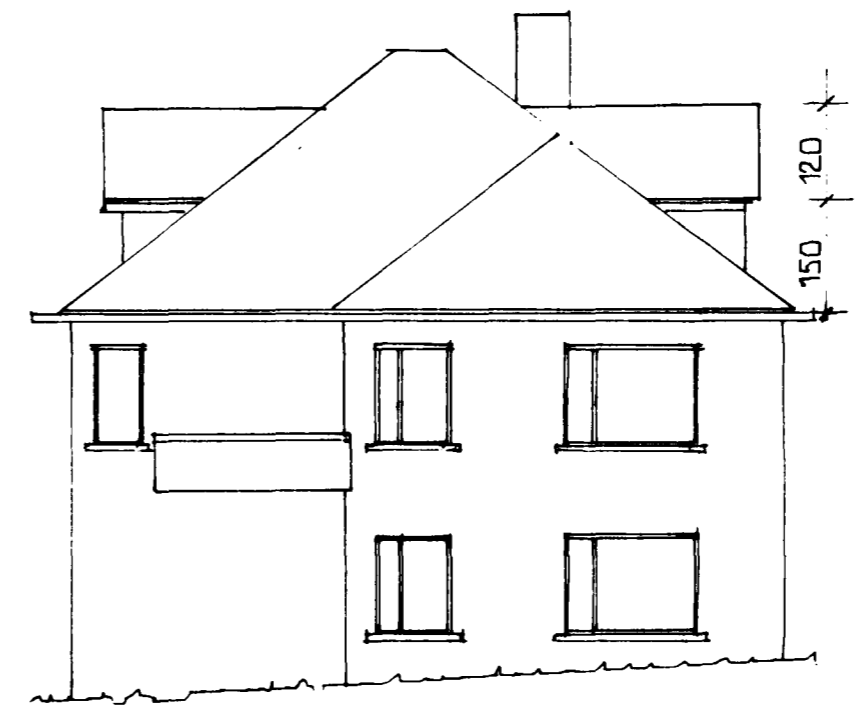
SUÐVESTUR
