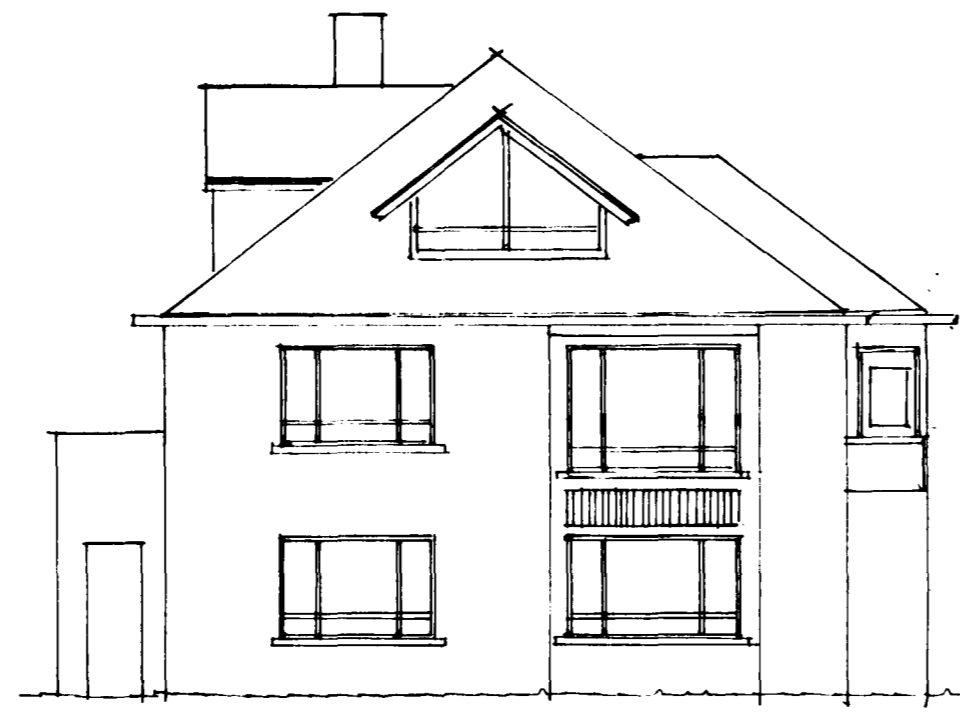
NORÐVESTUR
