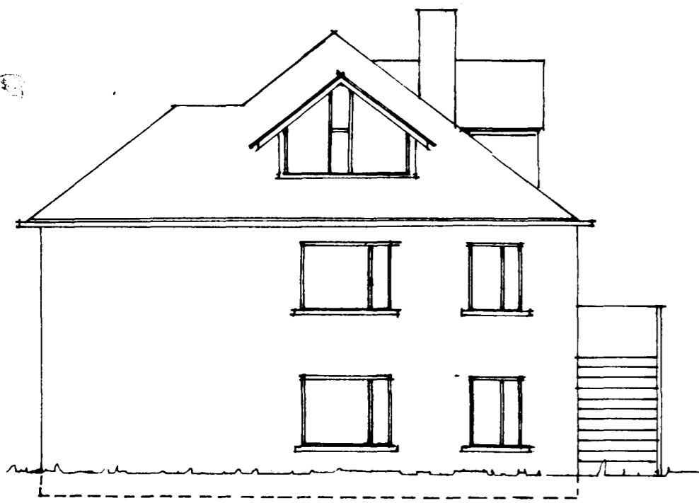
SUÐAUSTUR
