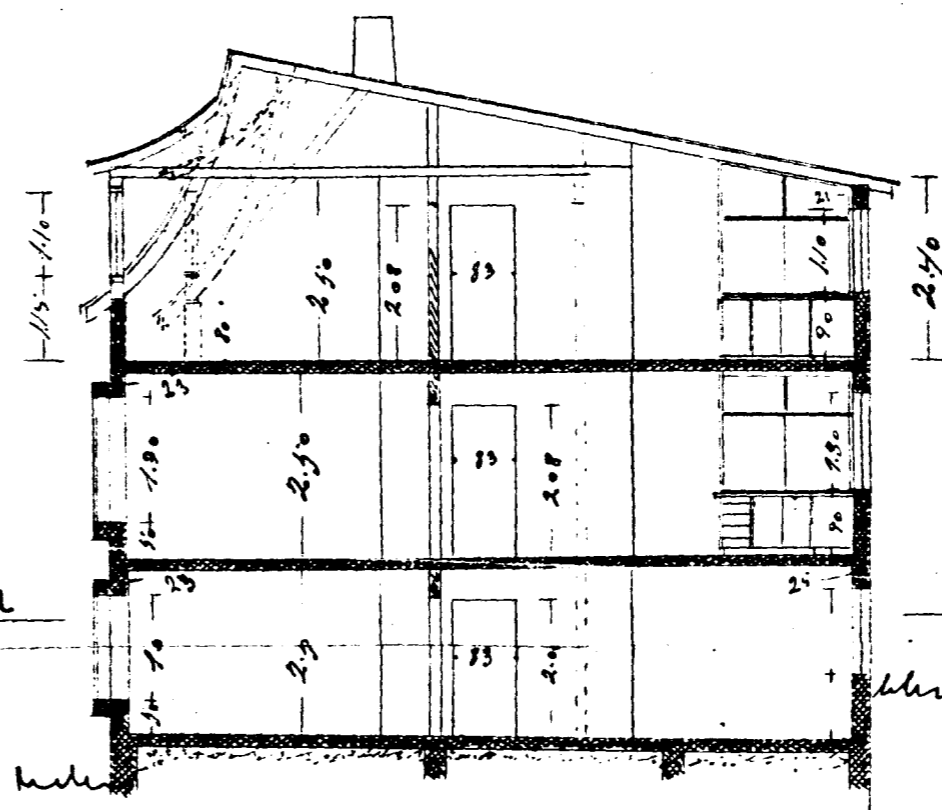
Þverskurður
