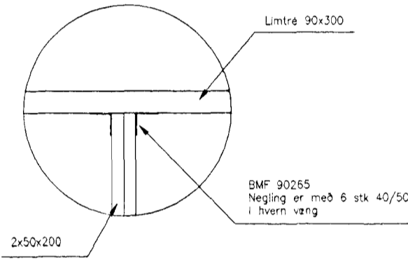
Snið nr 6
