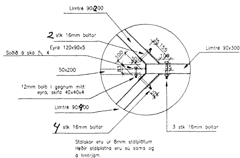
Snið nr 10
