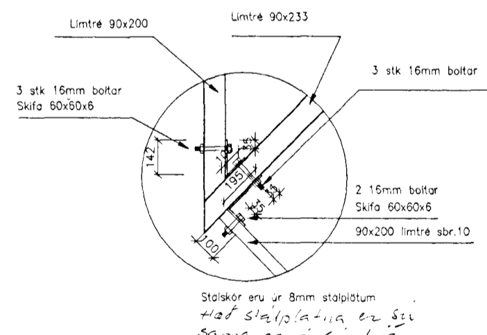
Snið nr 11
