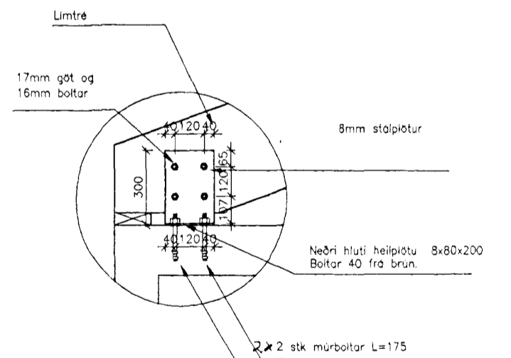
Snið nr 9
