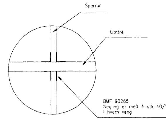
Snið nr 3
