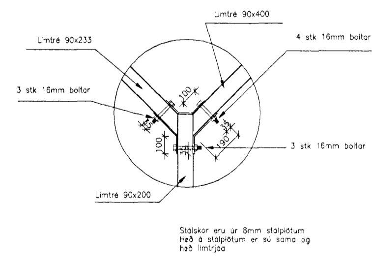
Snið nr 12
