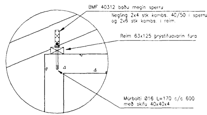
Snið nr 1
