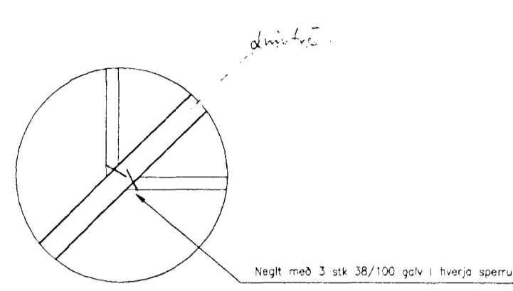
Snið nr 2
