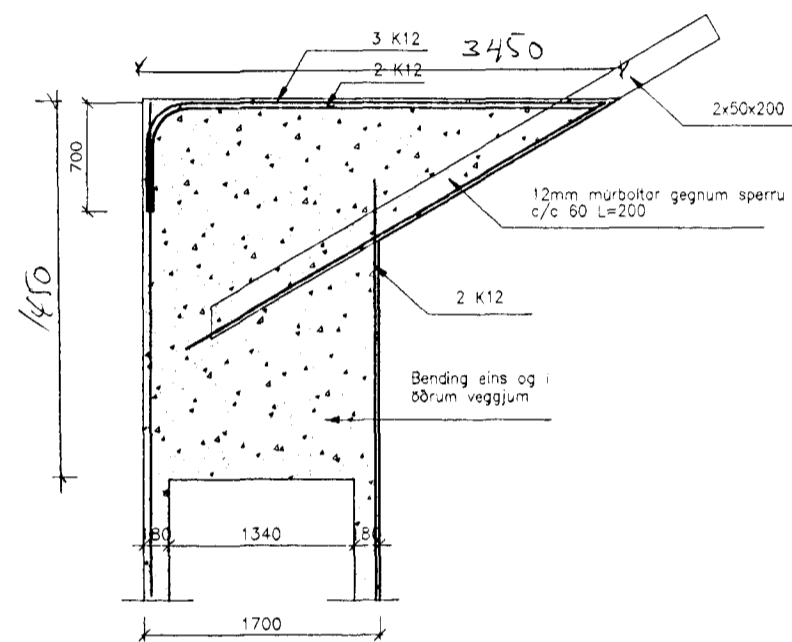
Snið nr 5 1:50
