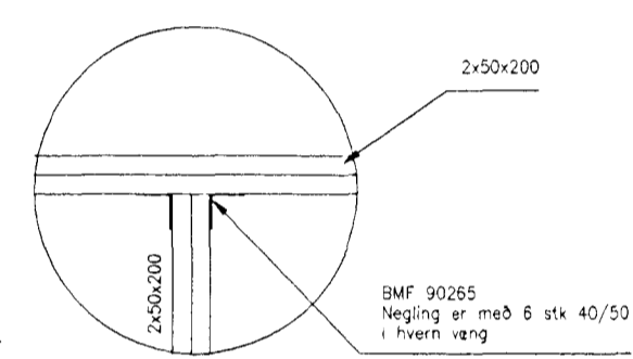
Snið nr 8
