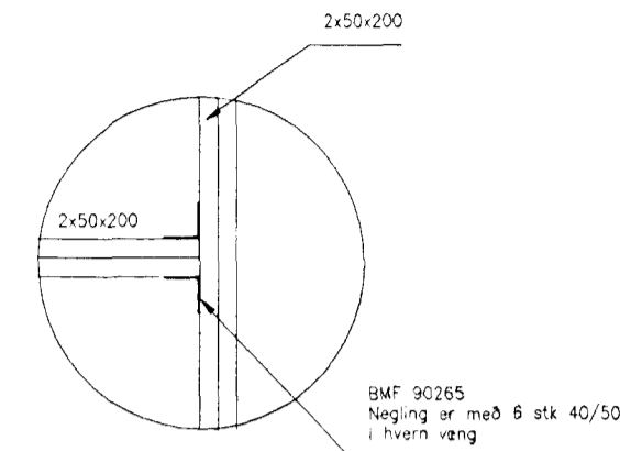
Snið nr 4
