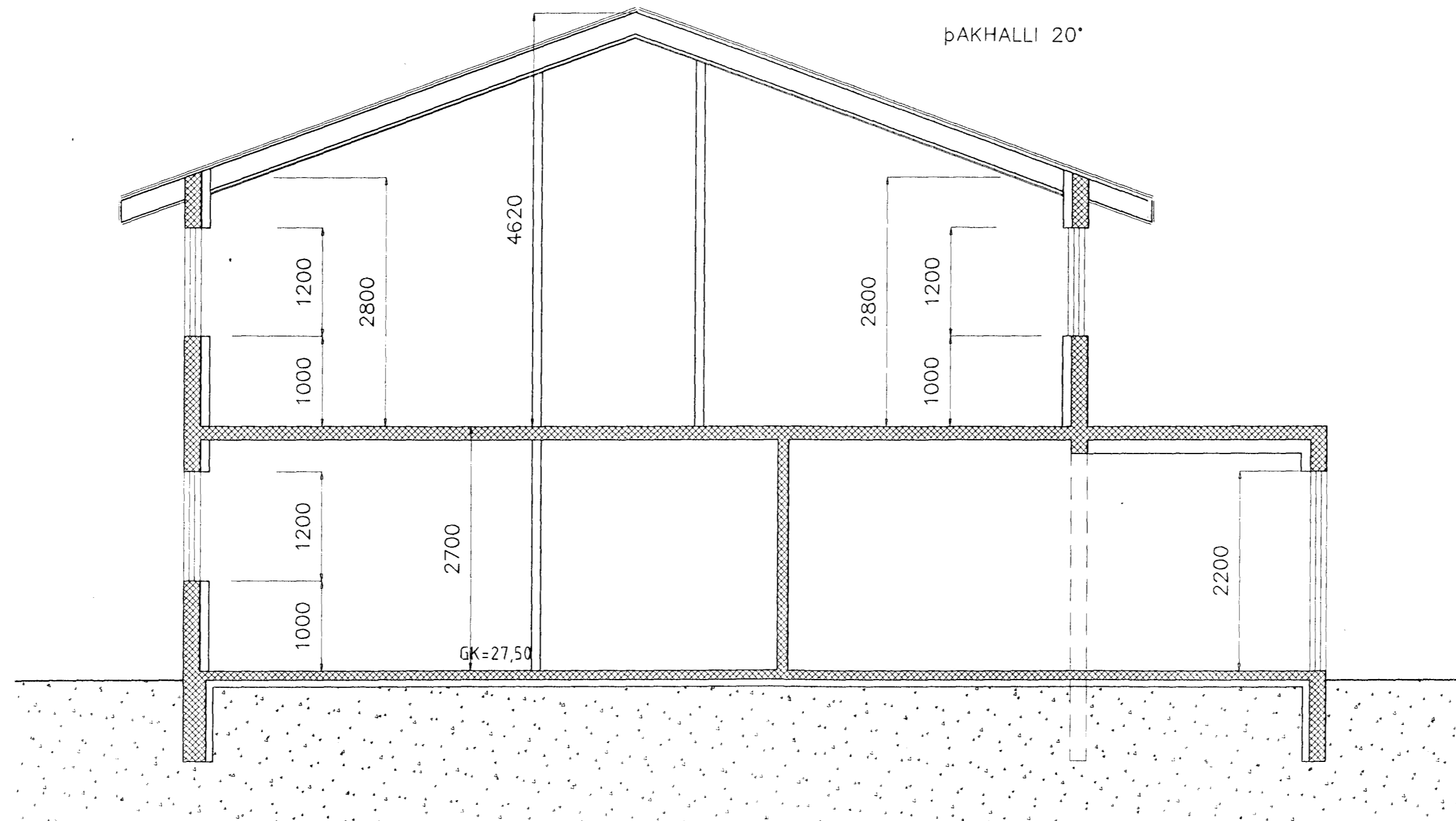
SNID A-A
