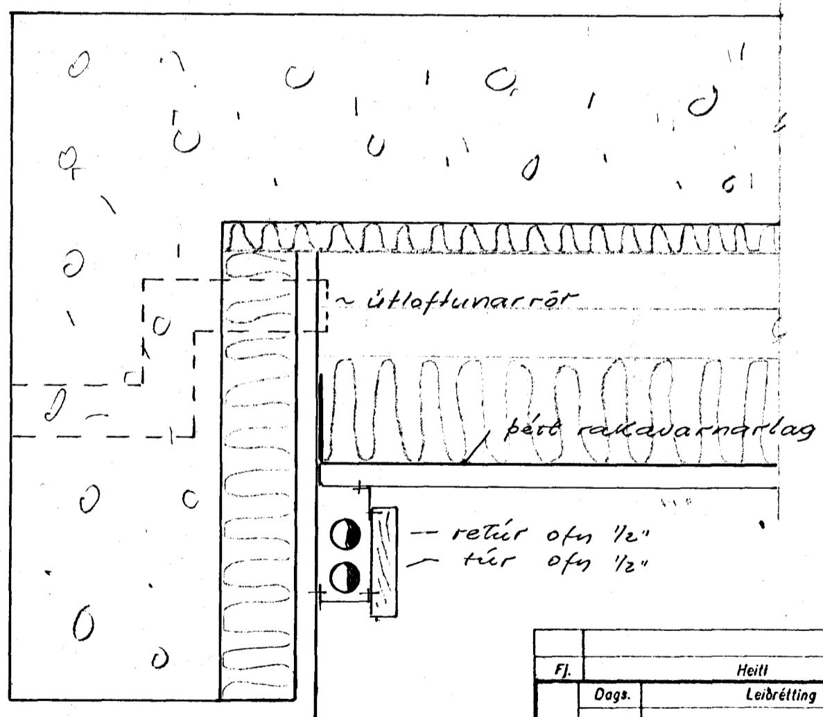
Skurður C-C MKV ~ 1:5
