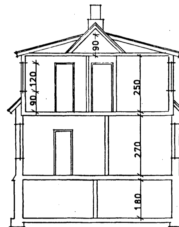
SKURÐMYND
