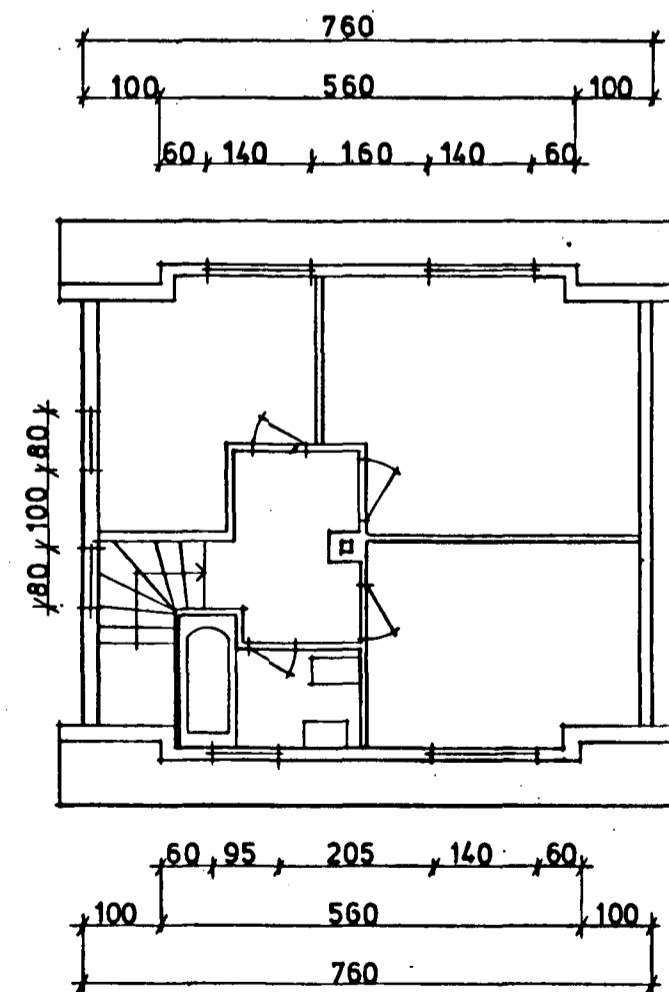
GRUNNMYND RISHÆÐAR
