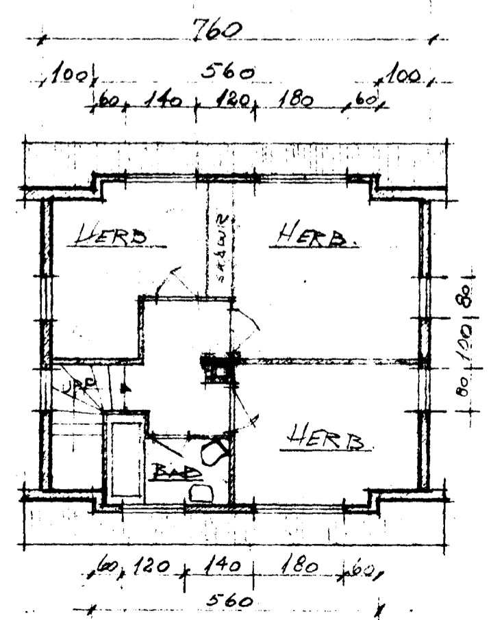
GRUNNMYND RISHED KVARDI 1:100
