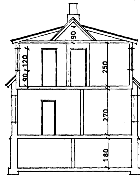
SKURÐMYND
