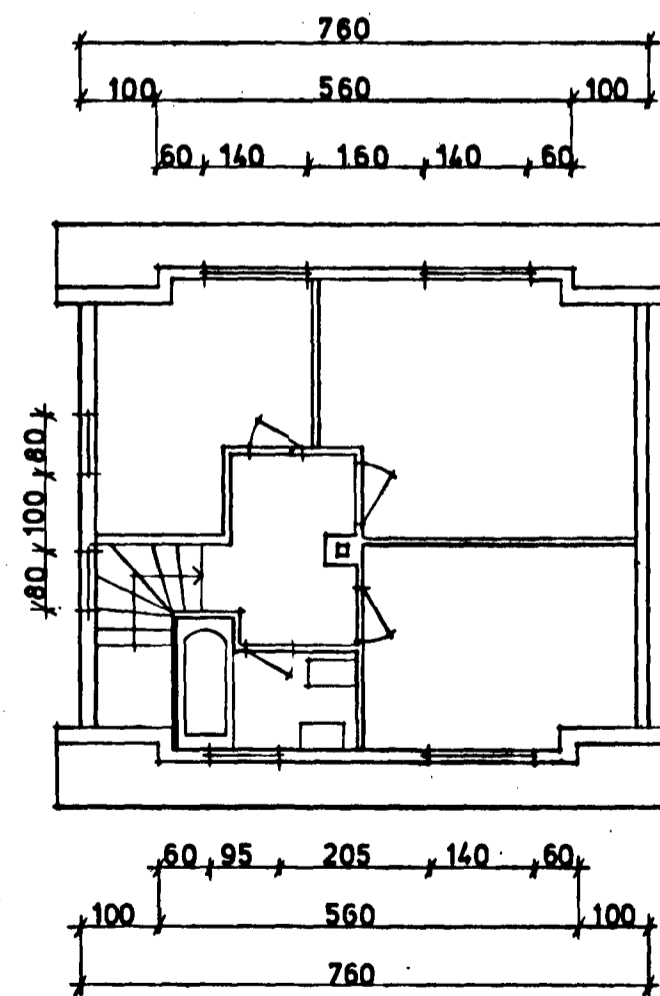
GRUNNMYND RISHÆÐAR
