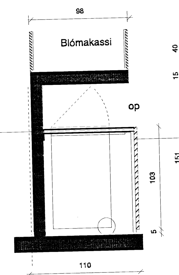
Snið í sorp geymslu
