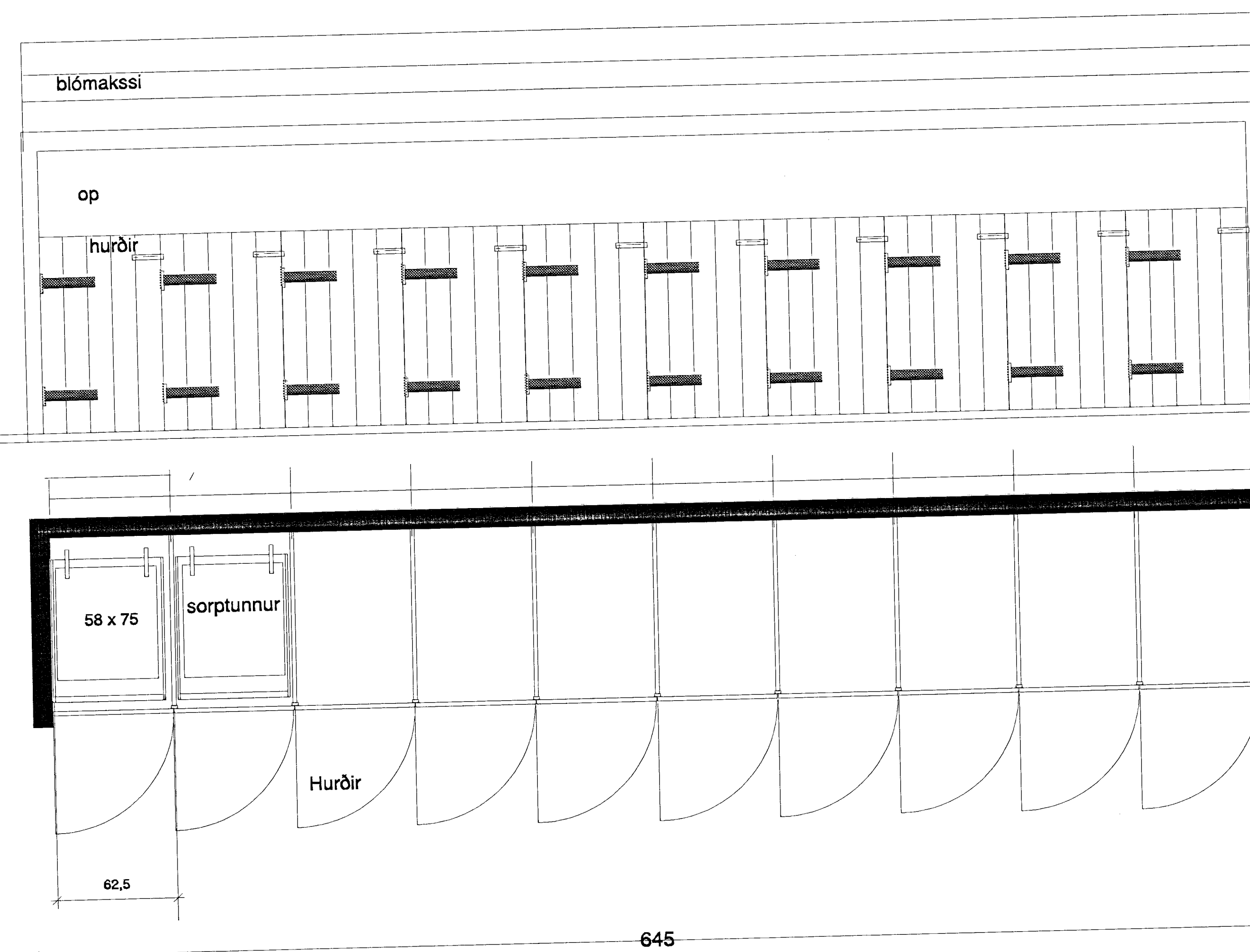
séð frama á sorpgeymslu
