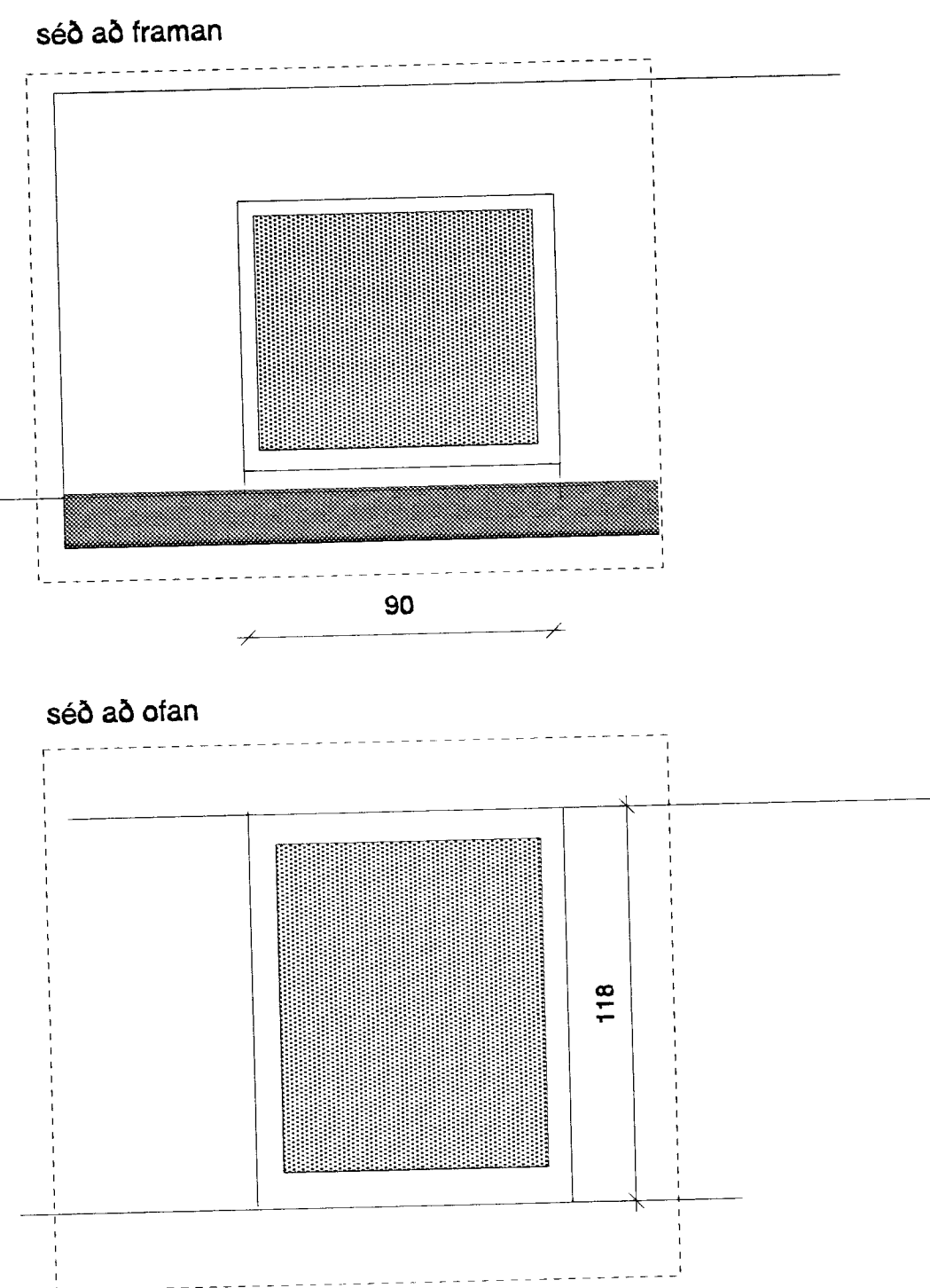
snið og útlit af glugga við geymslur 1 : 20
