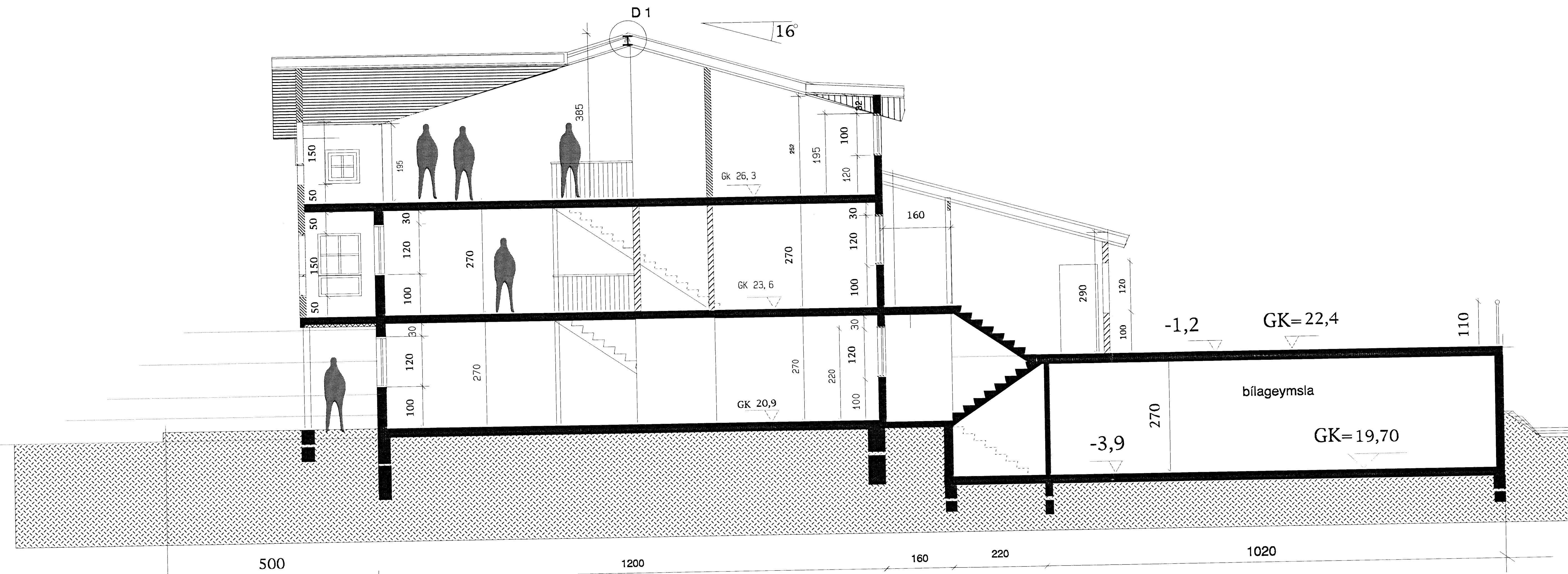
Snið A - A
