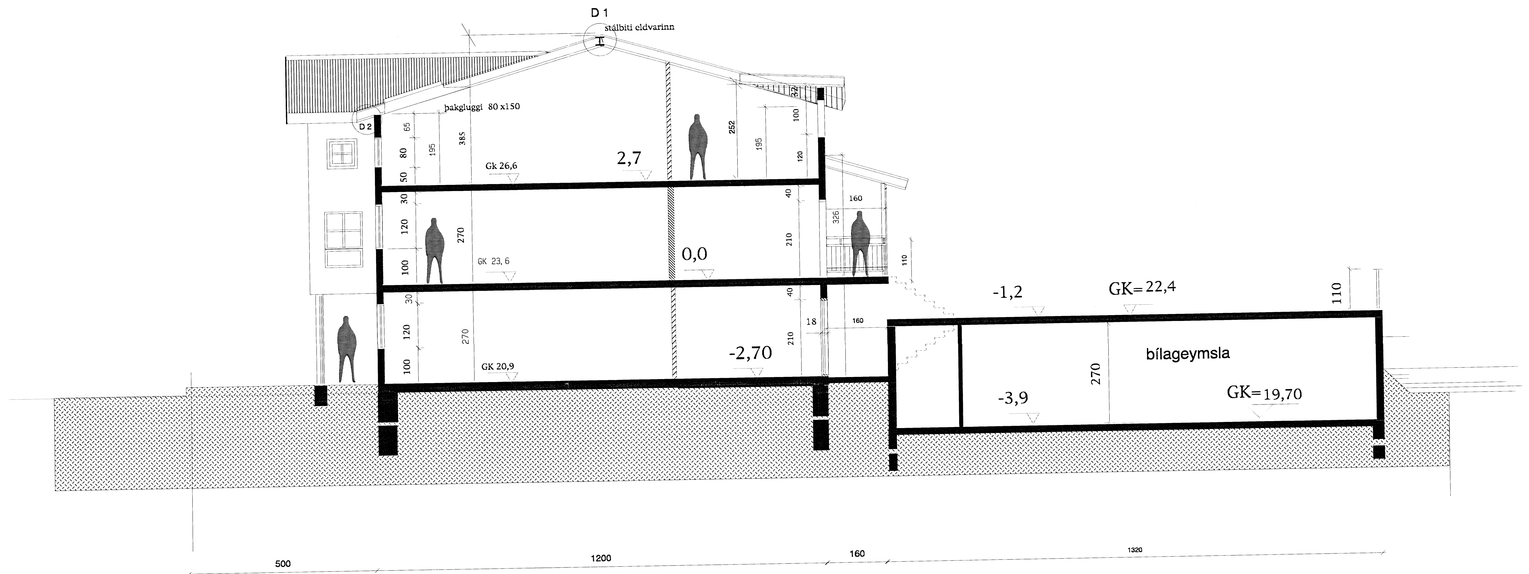
Snið B - B
