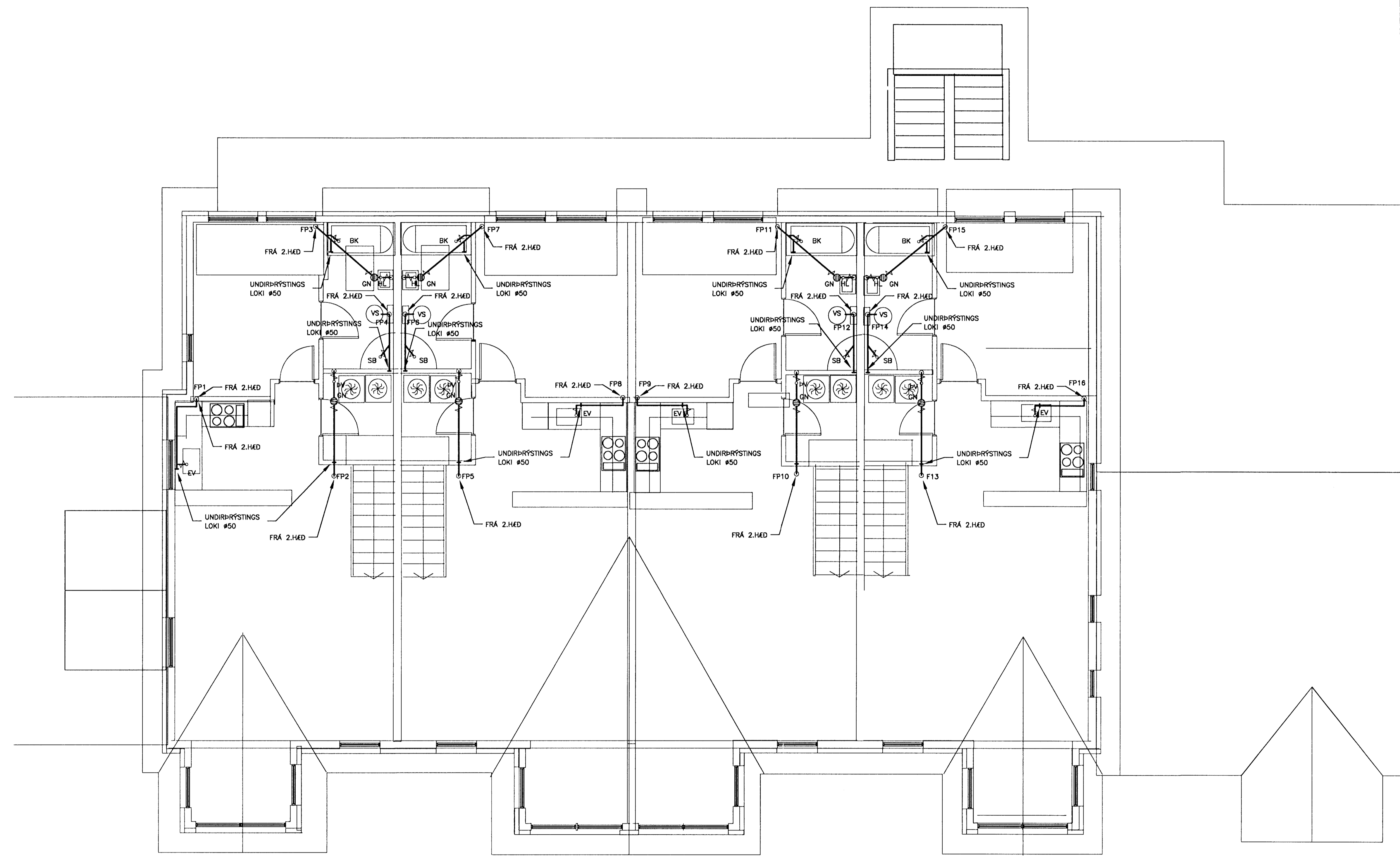
GRUNNMYND. 1:50
