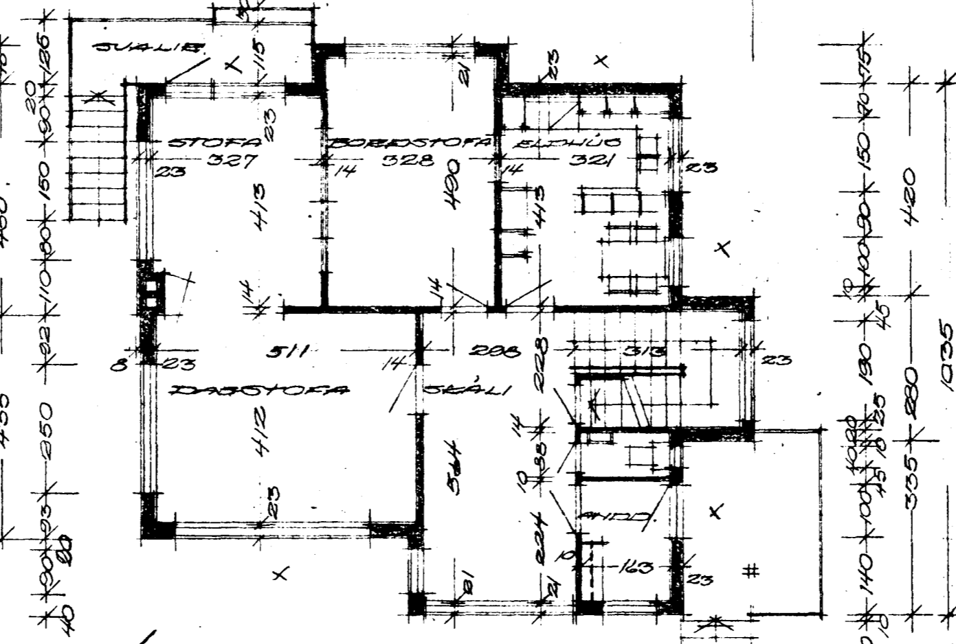
2. HÆÐ
