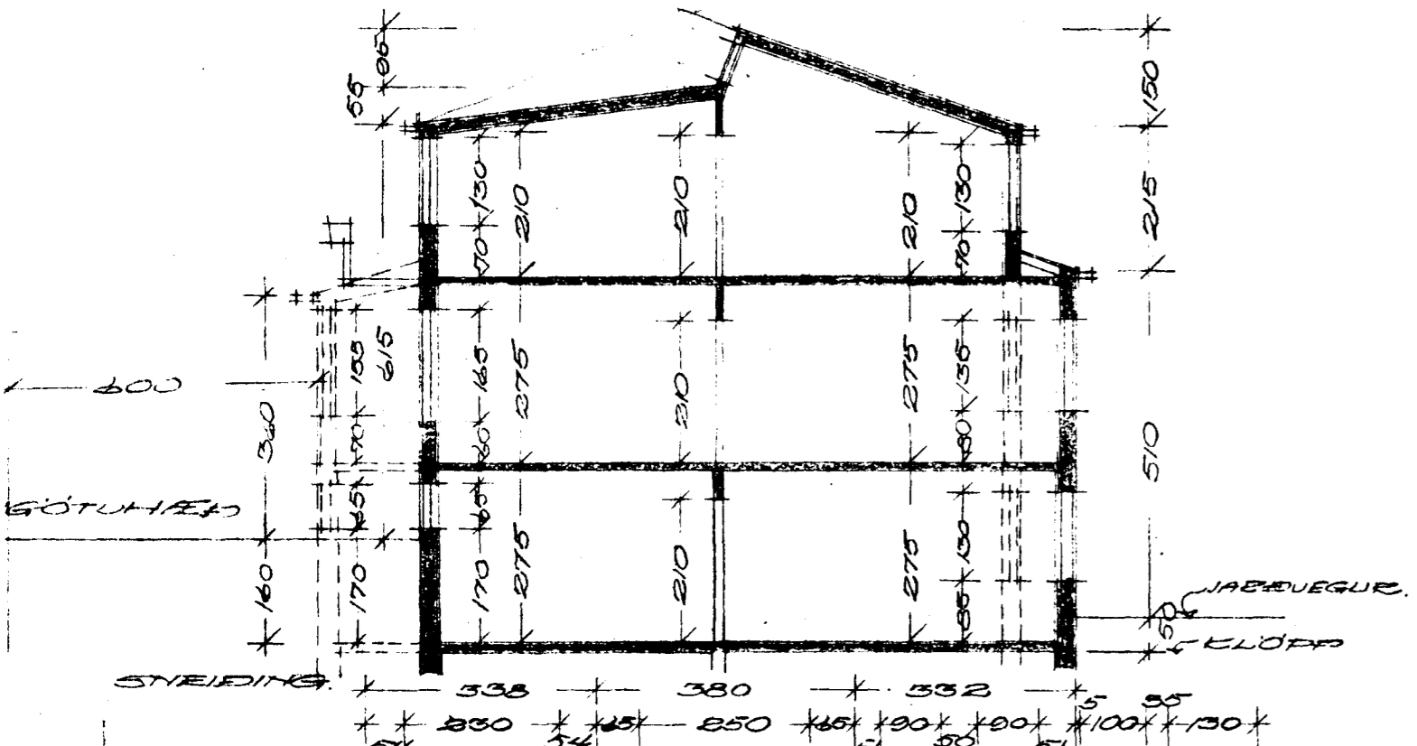
SÚÐURVESTUR.
