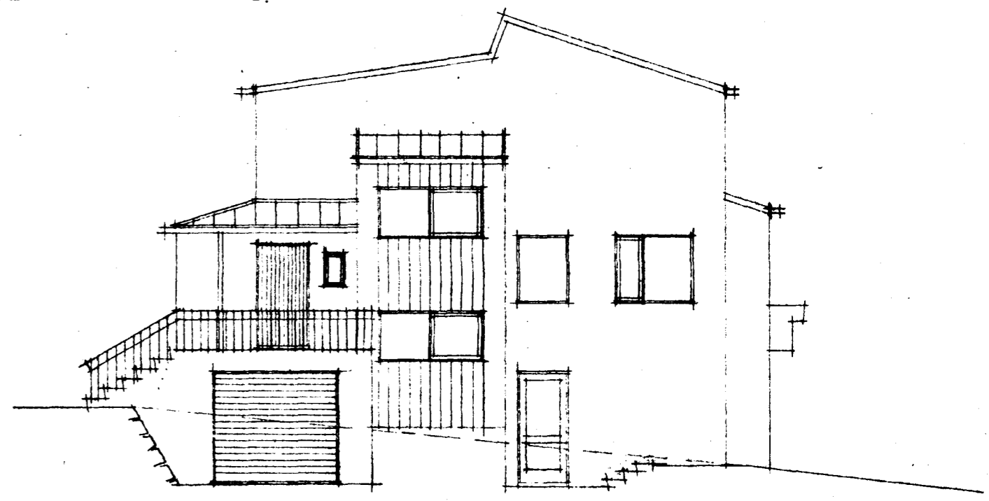
NOÐURAUÐTUSUR.
