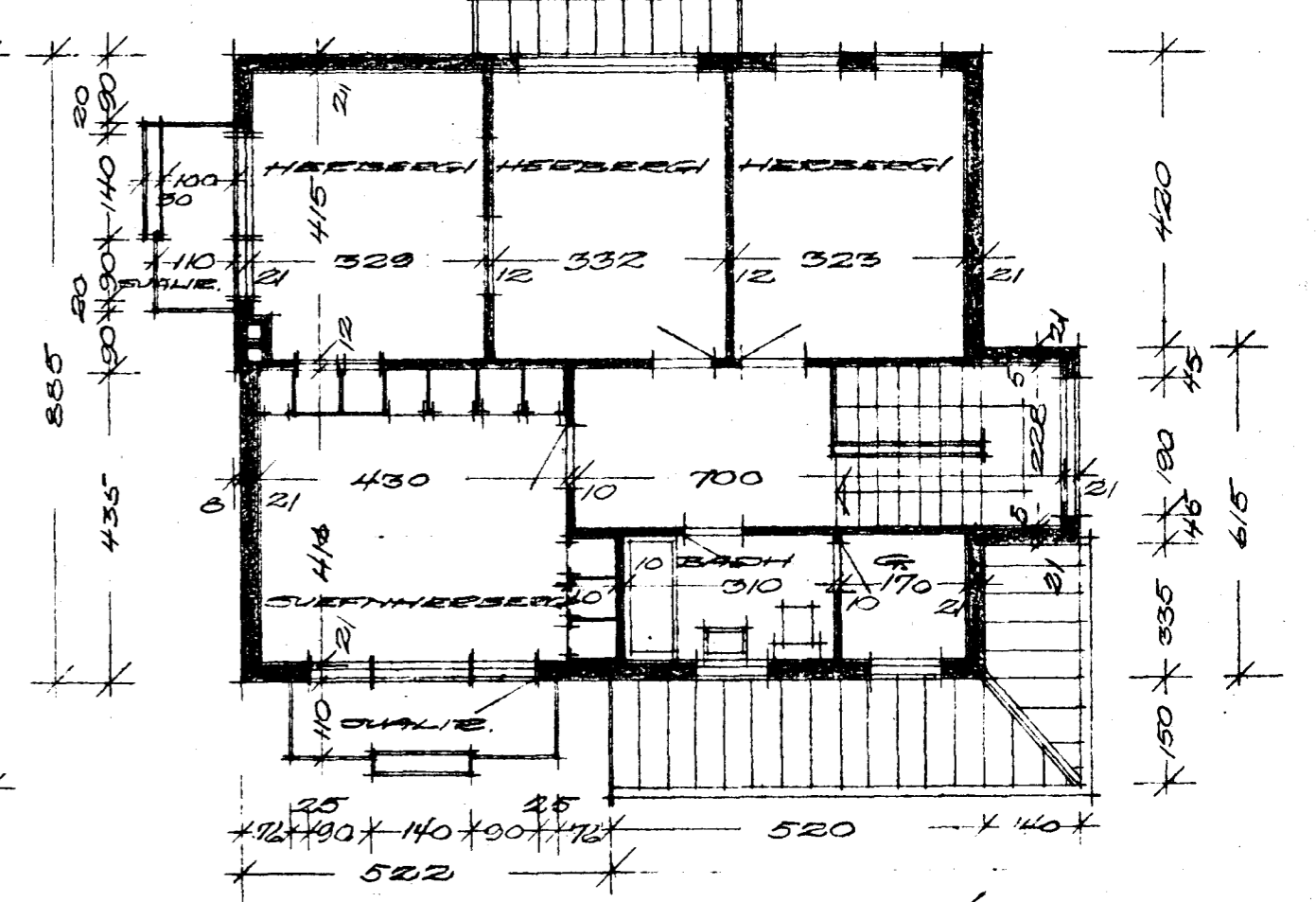
ÞAKHÆÐ.
