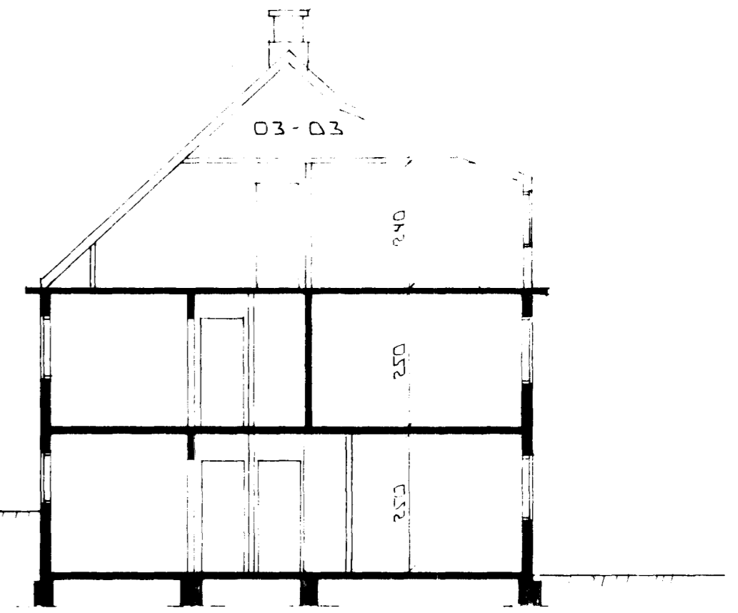
SNID A-A • 1:100
