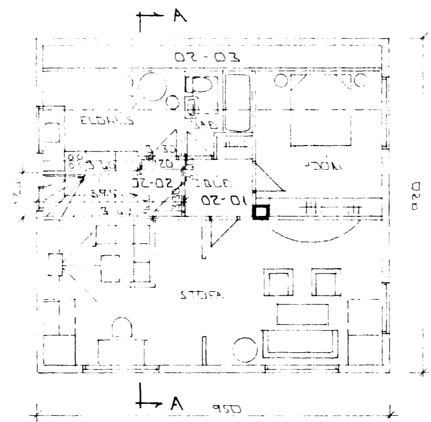
GRUNNMUND 2. HÆÐ • 1:100
