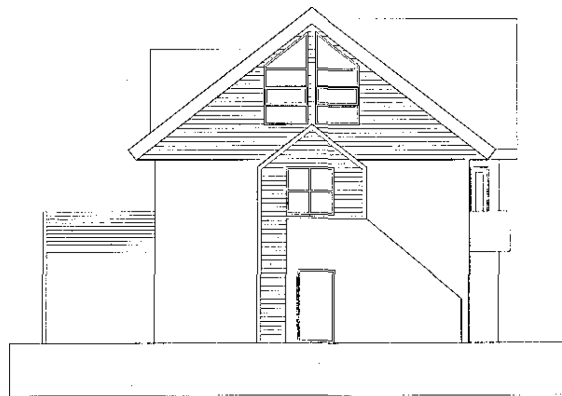
Útlit Norð-Austur 1:100
