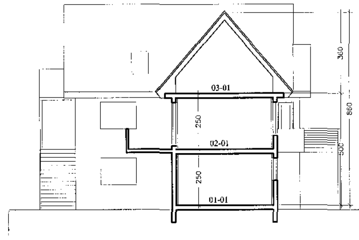
Sneiðing b-b 1:100
