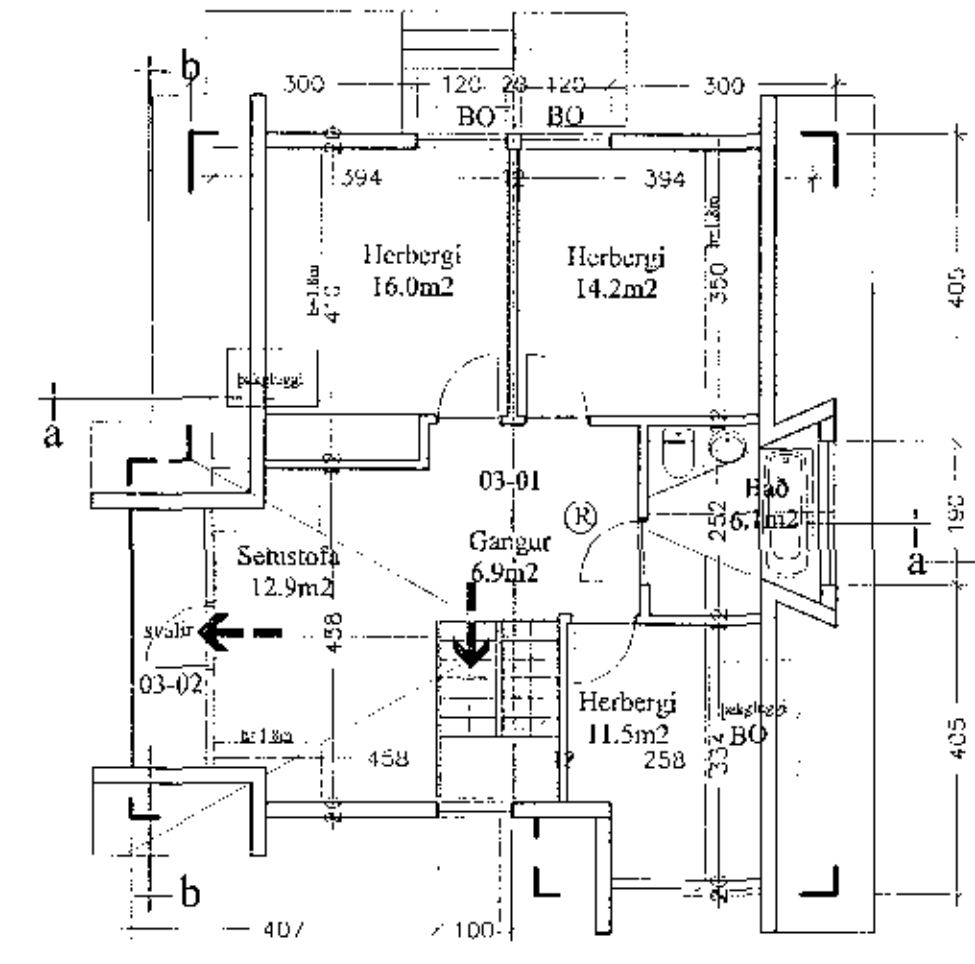
Grunnmynd 3.hæð 1:100
