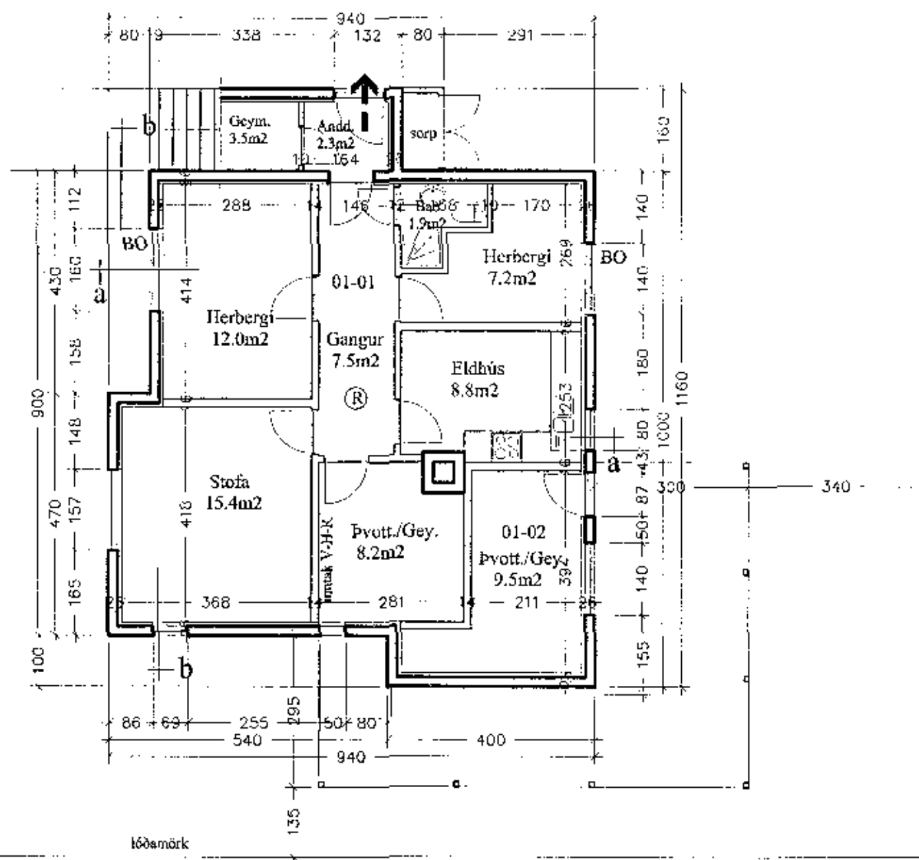
Grunnmynd 1.hæð 1:100
