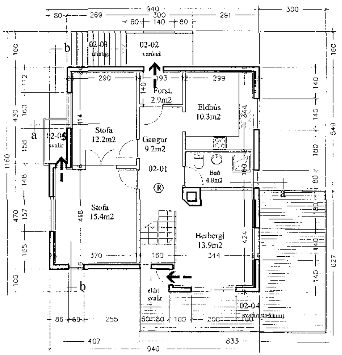
Grunnmynd 2.hæð 1:100
