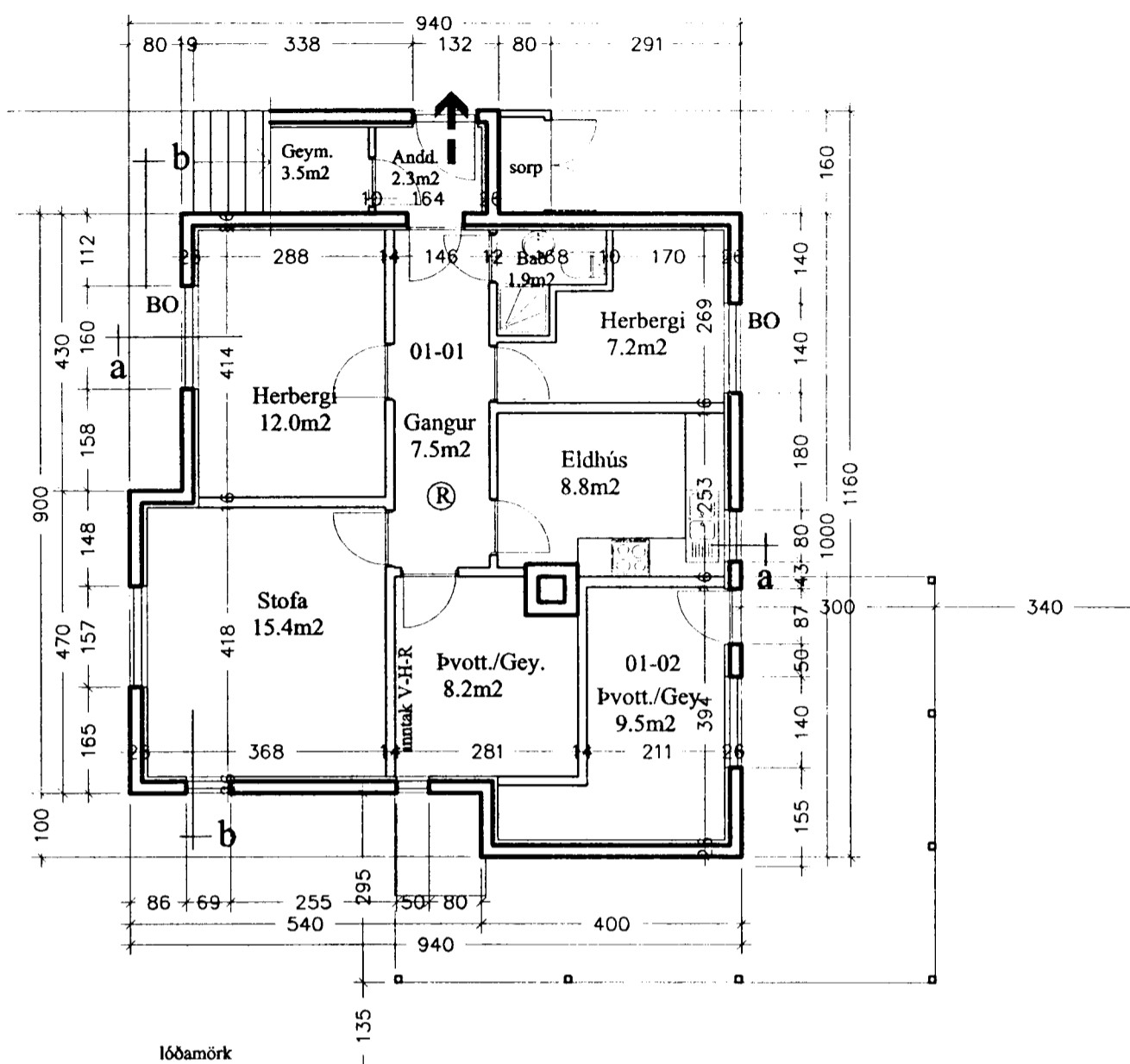
Grunnmynd 1.hæð 1:100
