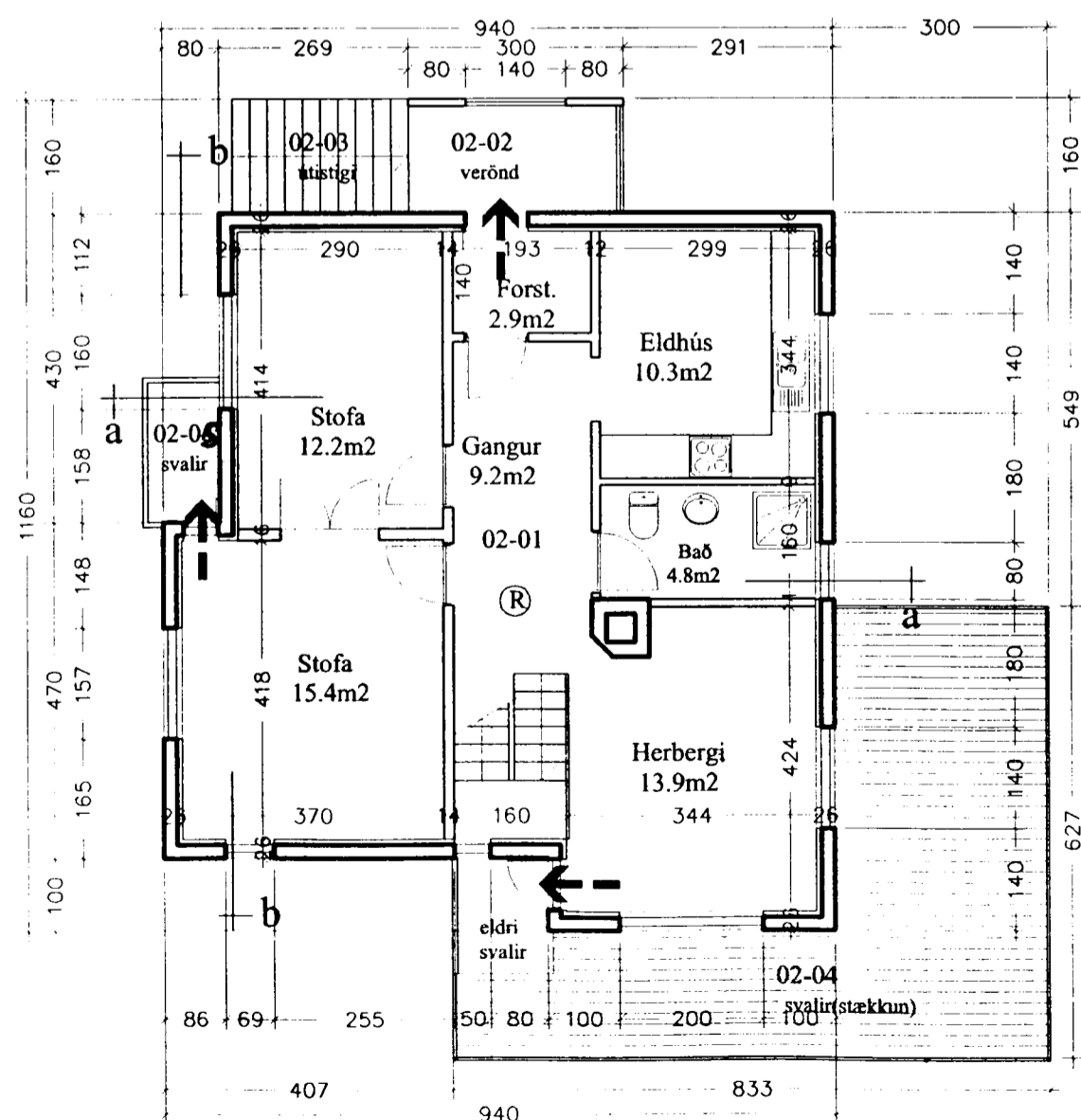
Grunnmynd 2.hæð 1:100
