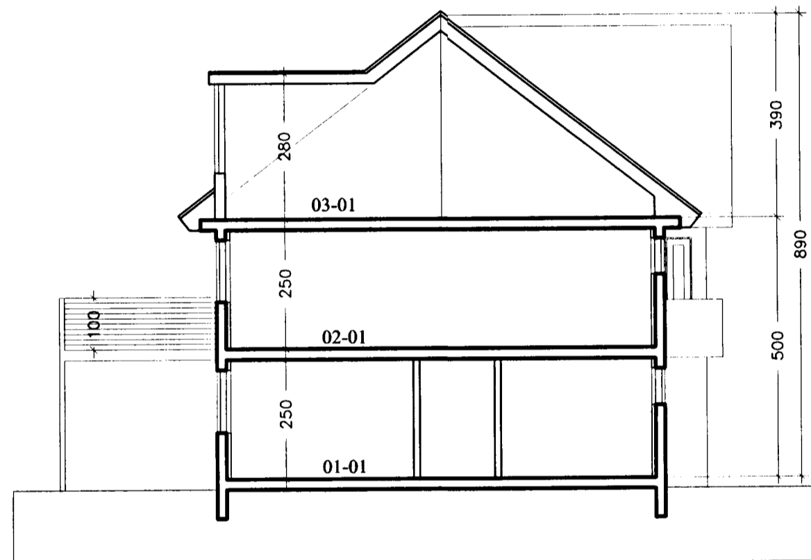
Sneiðing a-a 1:100
