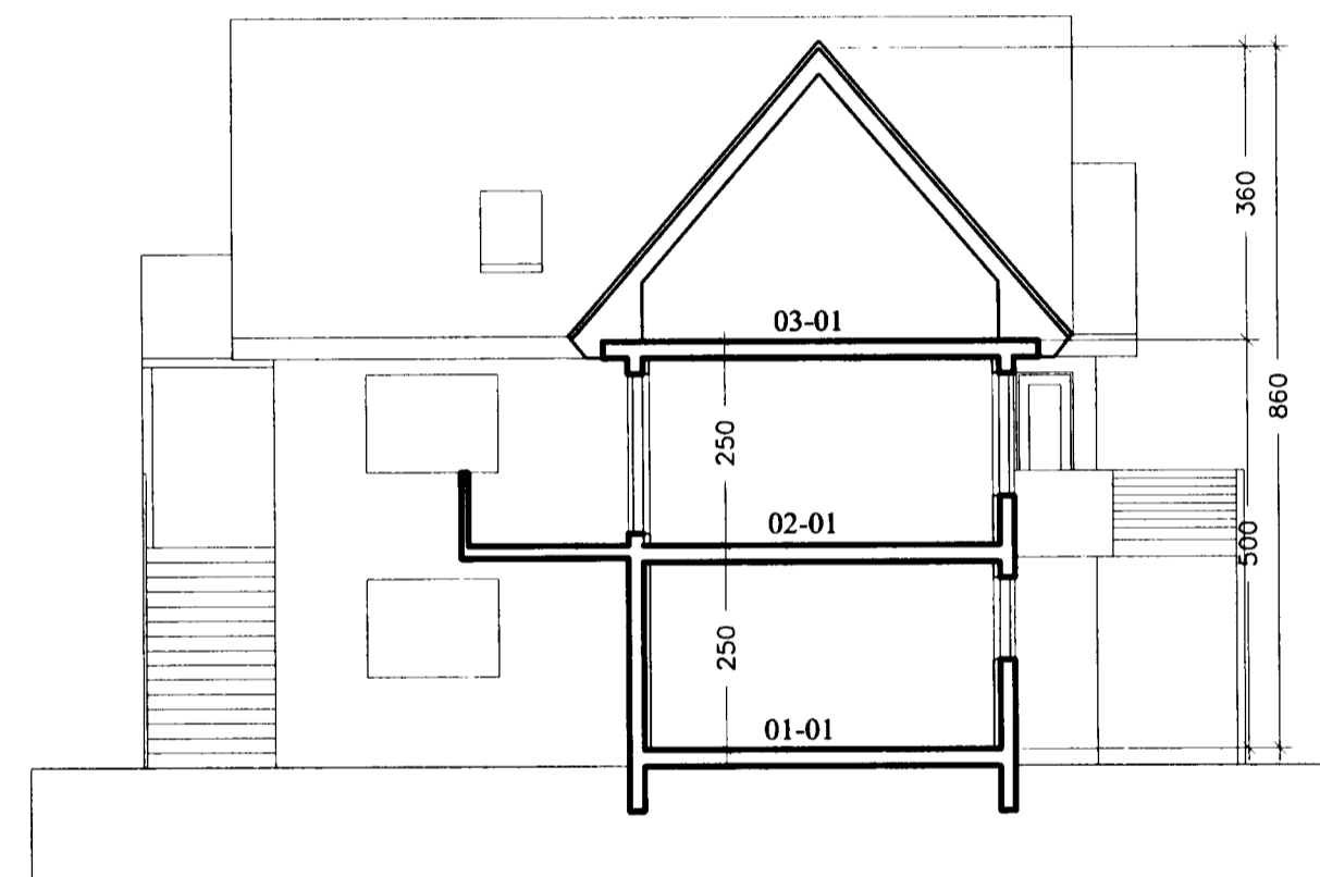
Sneiðing b-b 1:100
