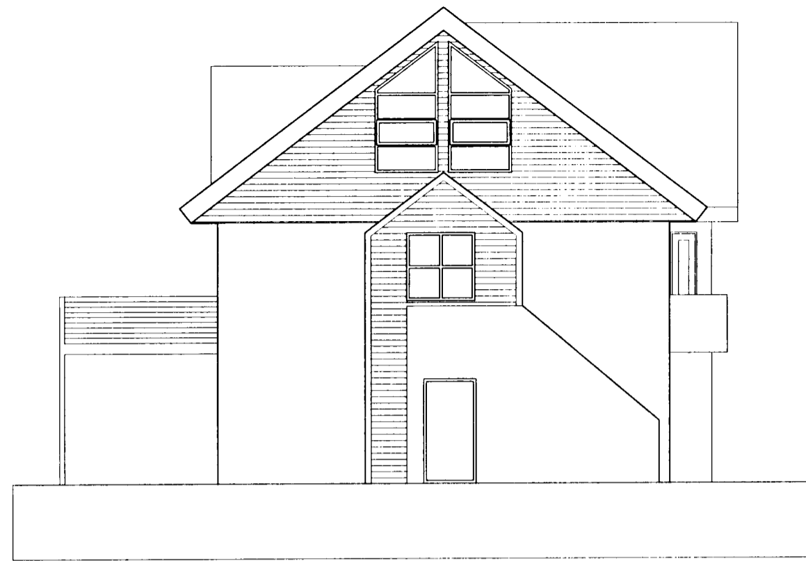
Útlit Norð-Austur 1:100
