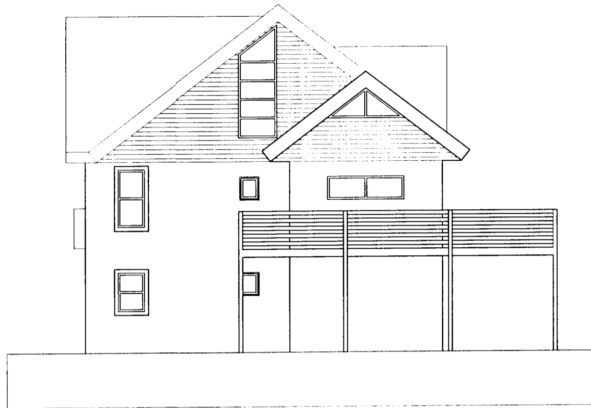
Útlit Suð-Vestur 1:100
