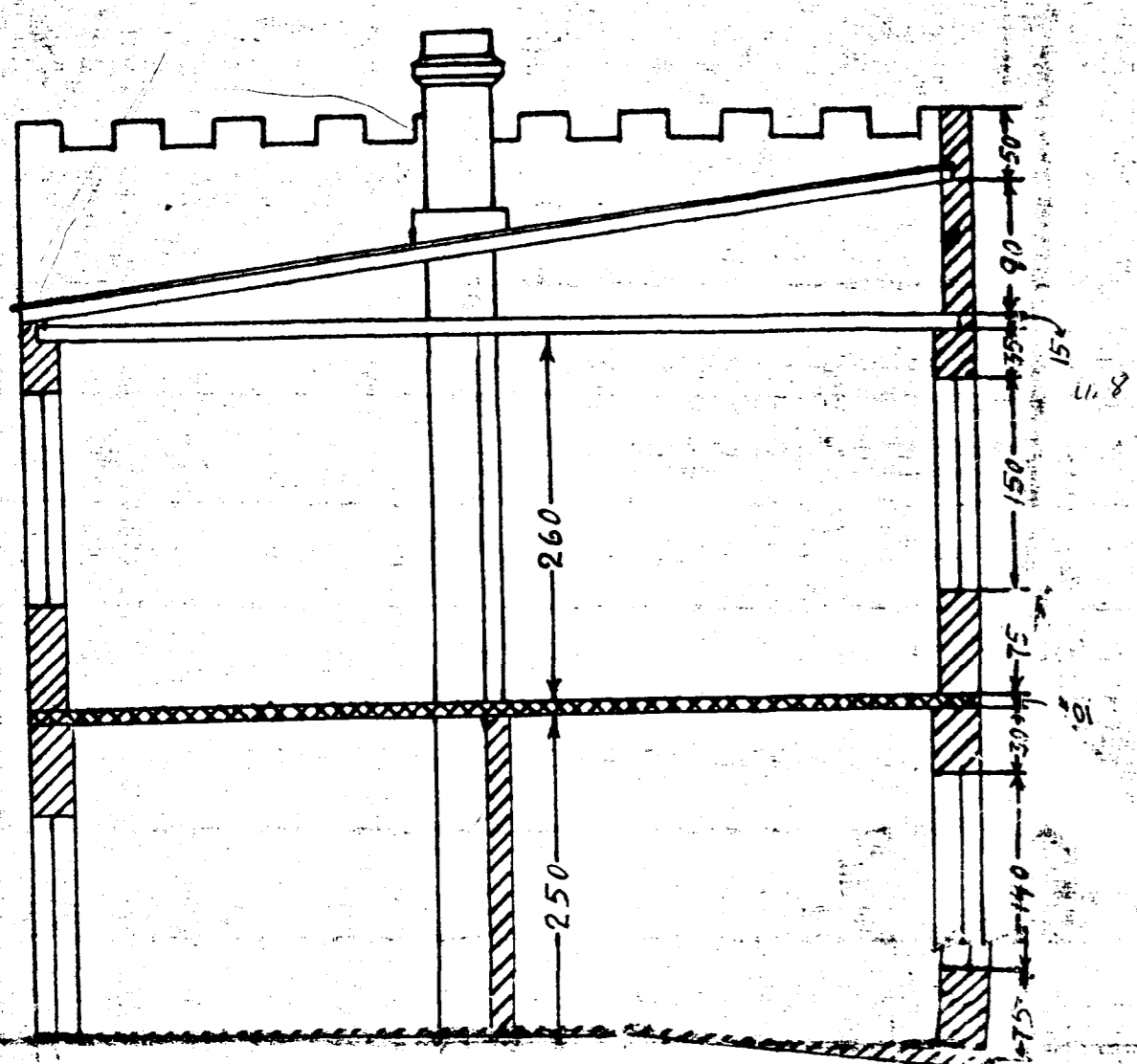
Kjallari
