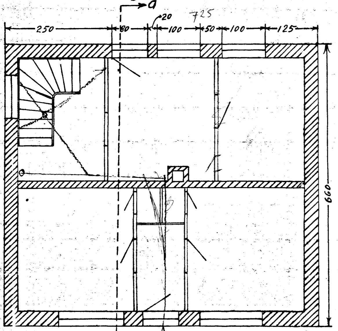
Kjallari
