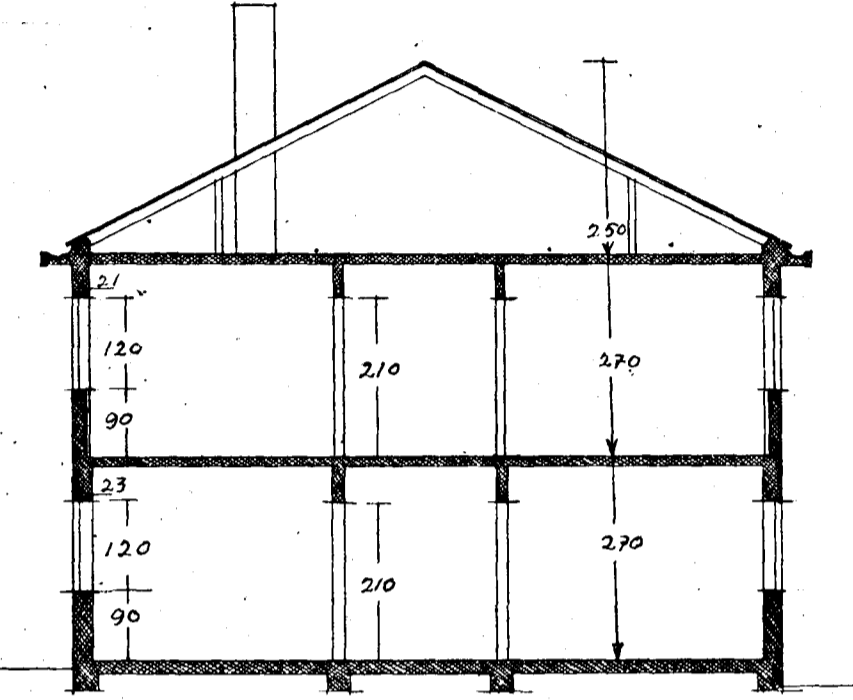
Snéiðing.
