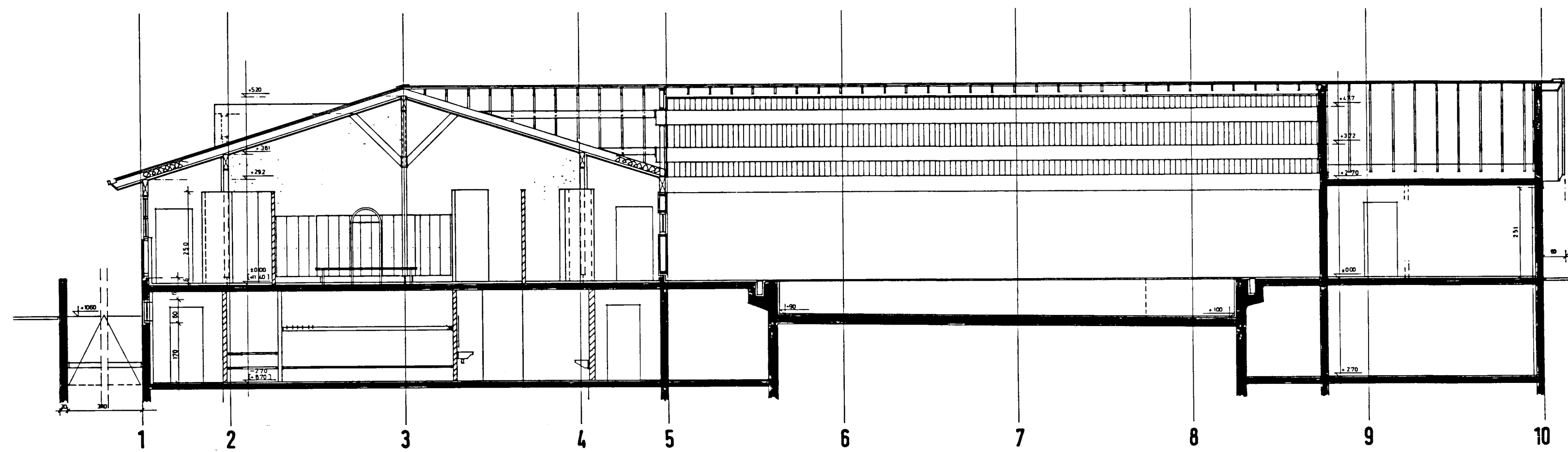
sneiding a-a
