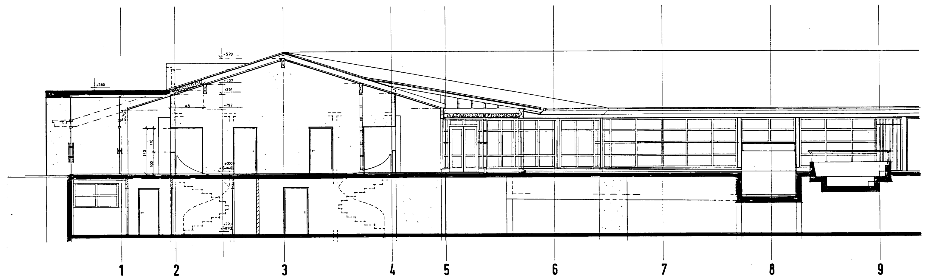
sneiding b-b
