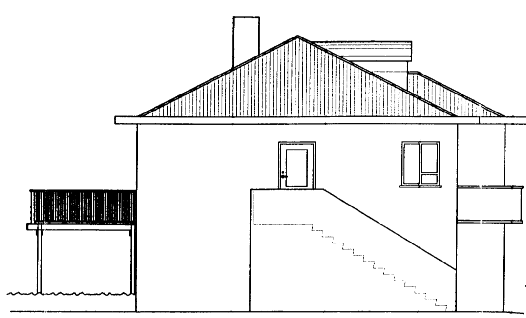
Útlit austurhlíð 1:100
