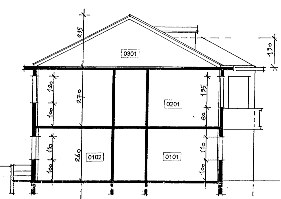
Sneiðing 1:100
