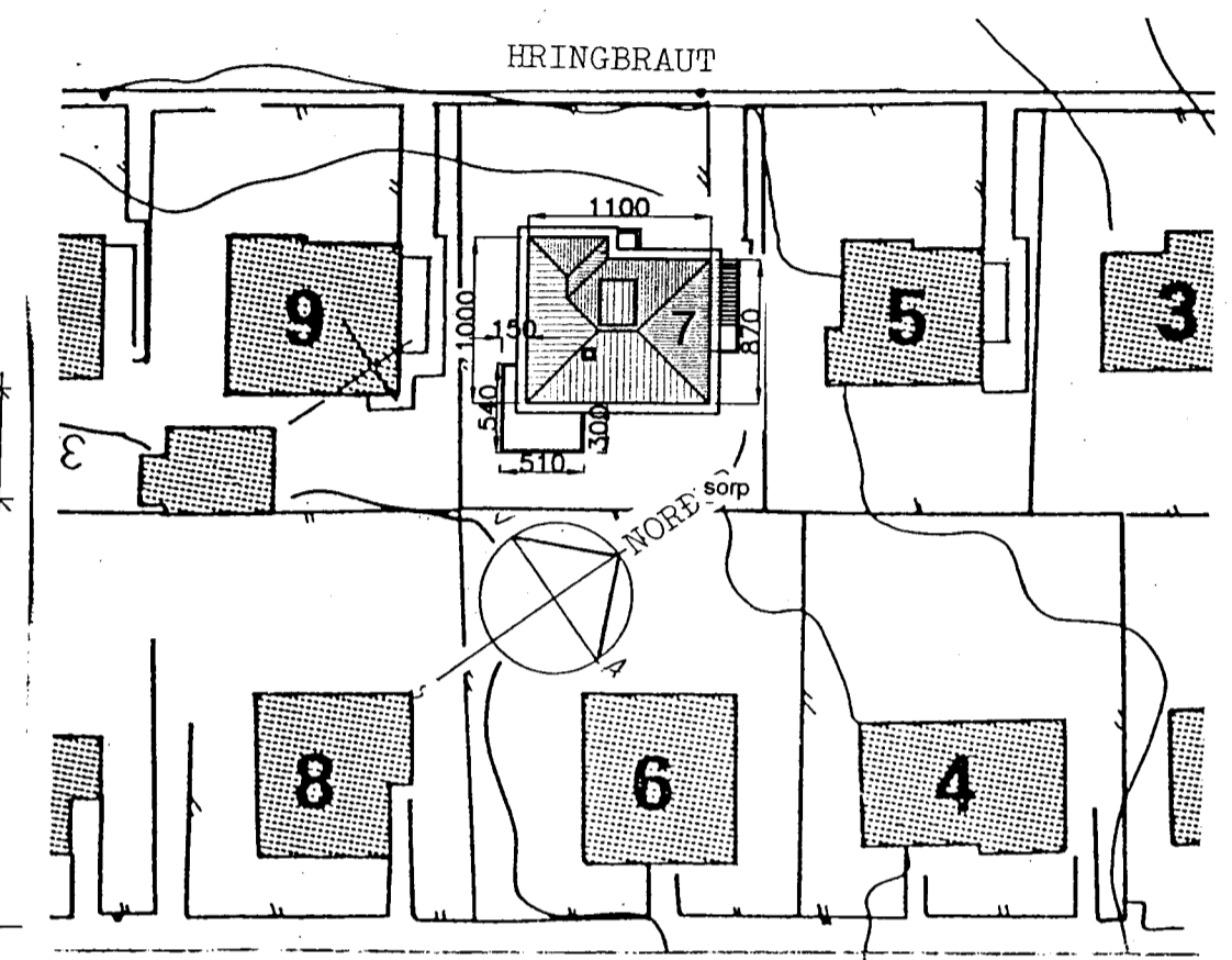
Afstöðumynd 1:500
