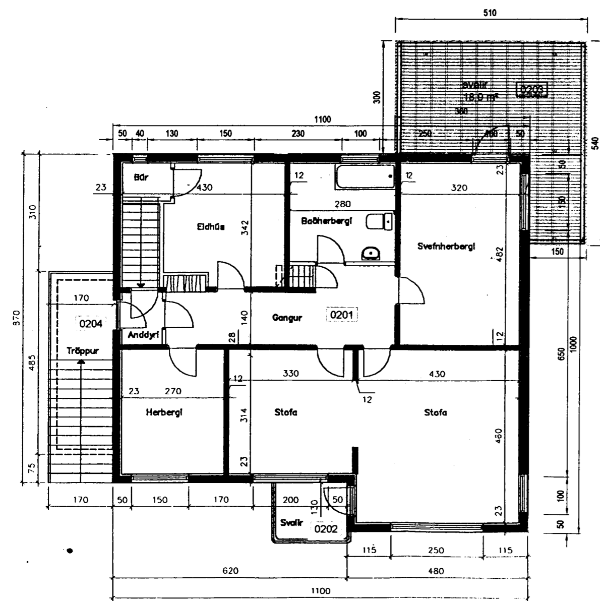
Grunnmynd efri hæðar 1:100
