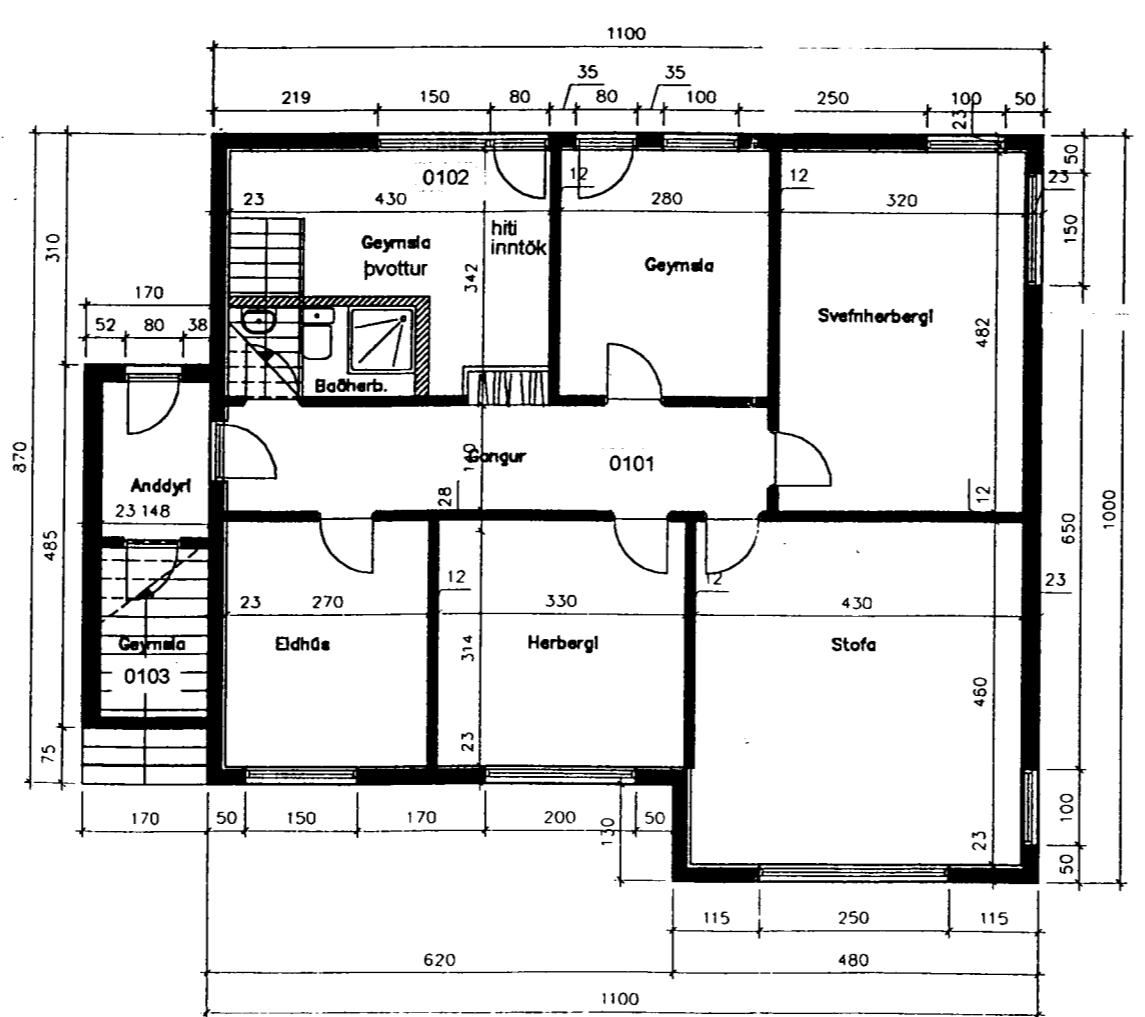
Grunnmynd neðri hæðar 1:100
