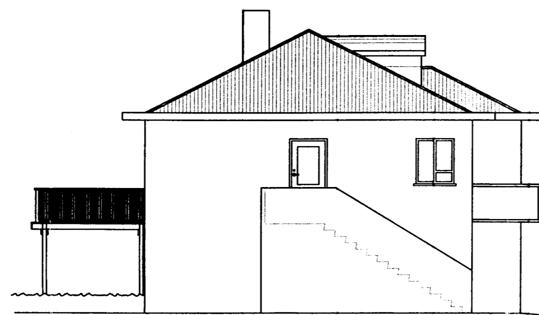
Útlit austurhlíð 1:100
