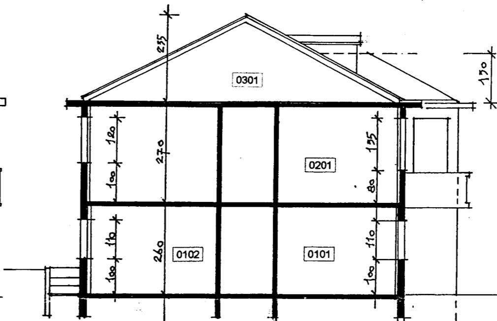
Sneiðing 1:100
