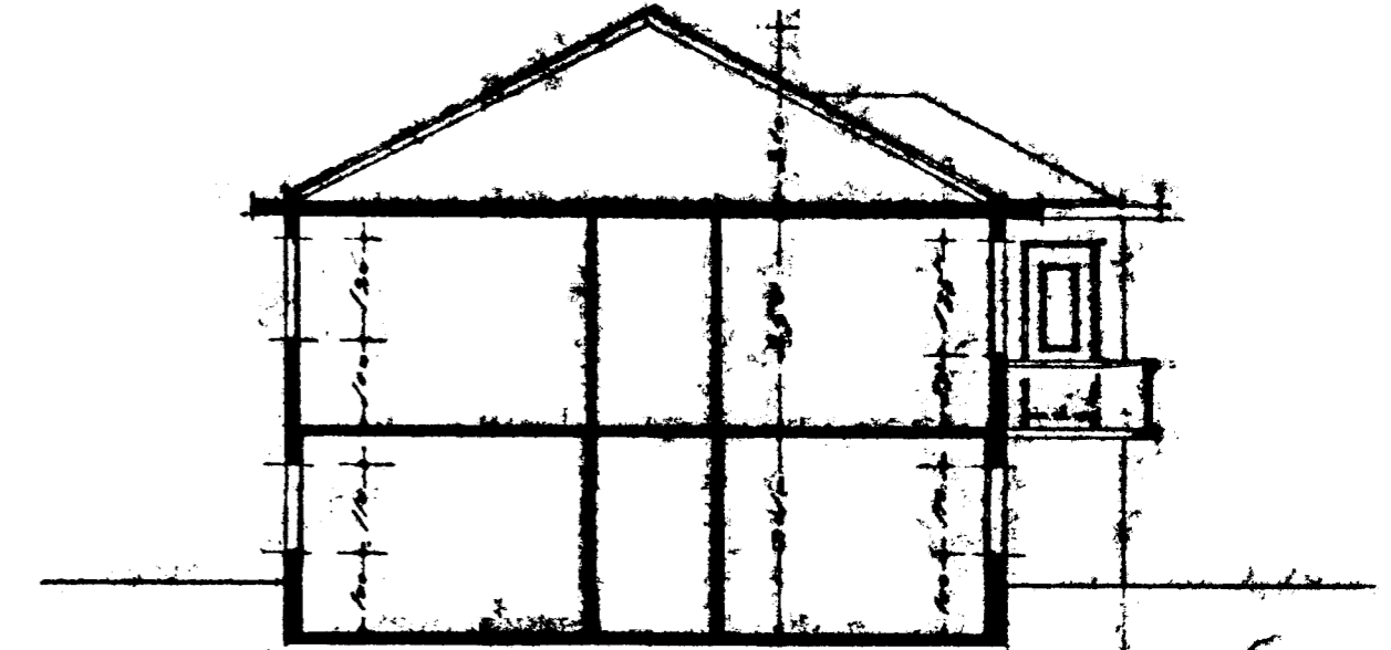
Skurður A-A
