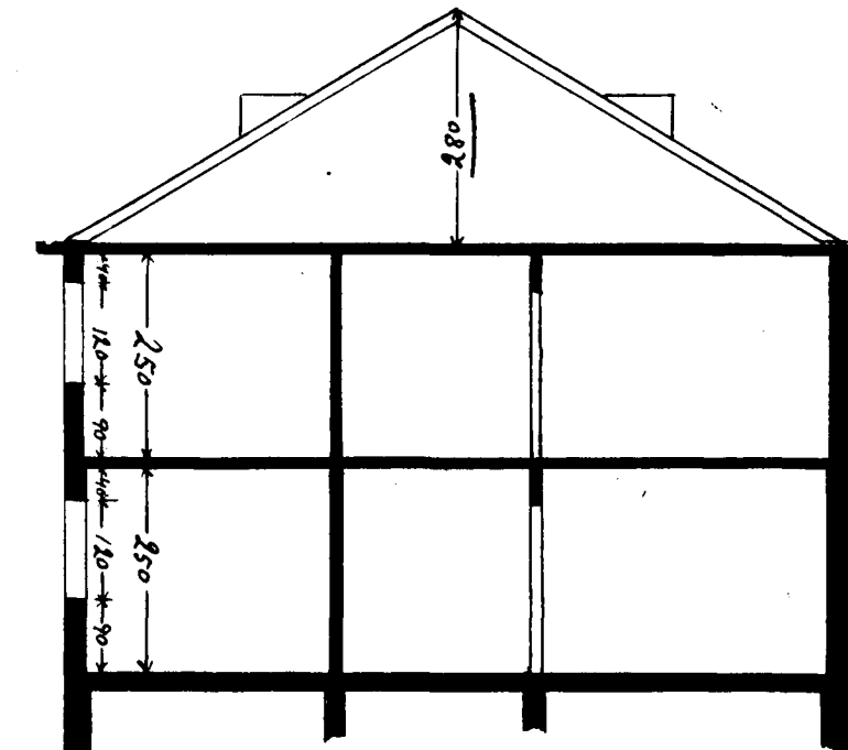
Skurður a-a
