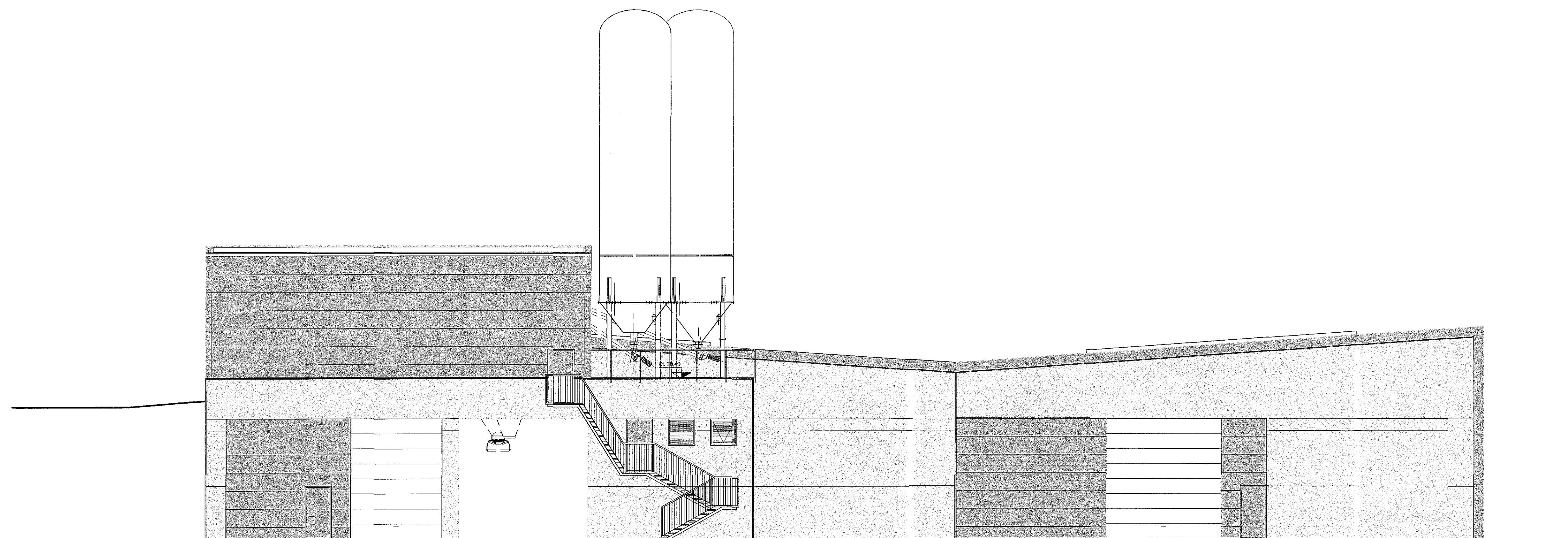
ÚTLIT AUSTUR
