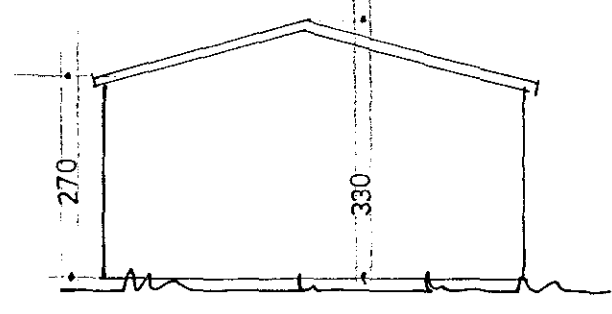
vestur gafi 1:100
