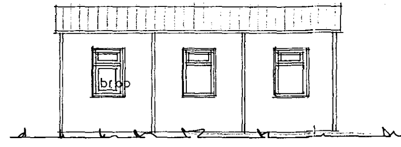
útlit nordur 1:100
