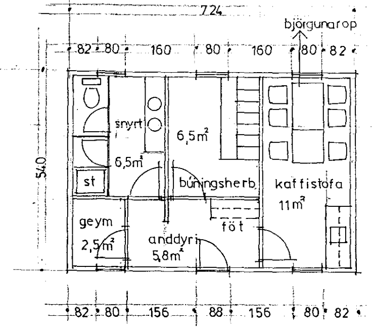
grunnmynd 1:100
