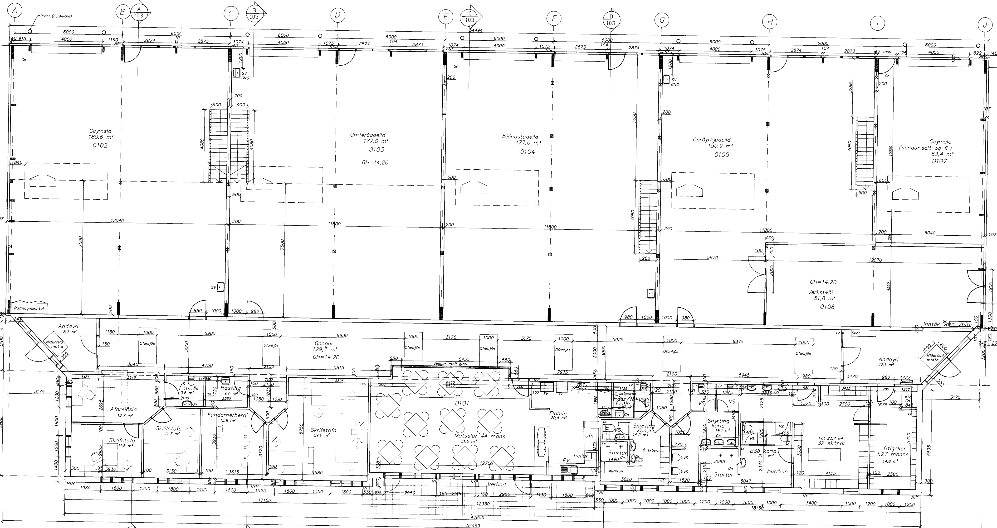
Grunnmynd
