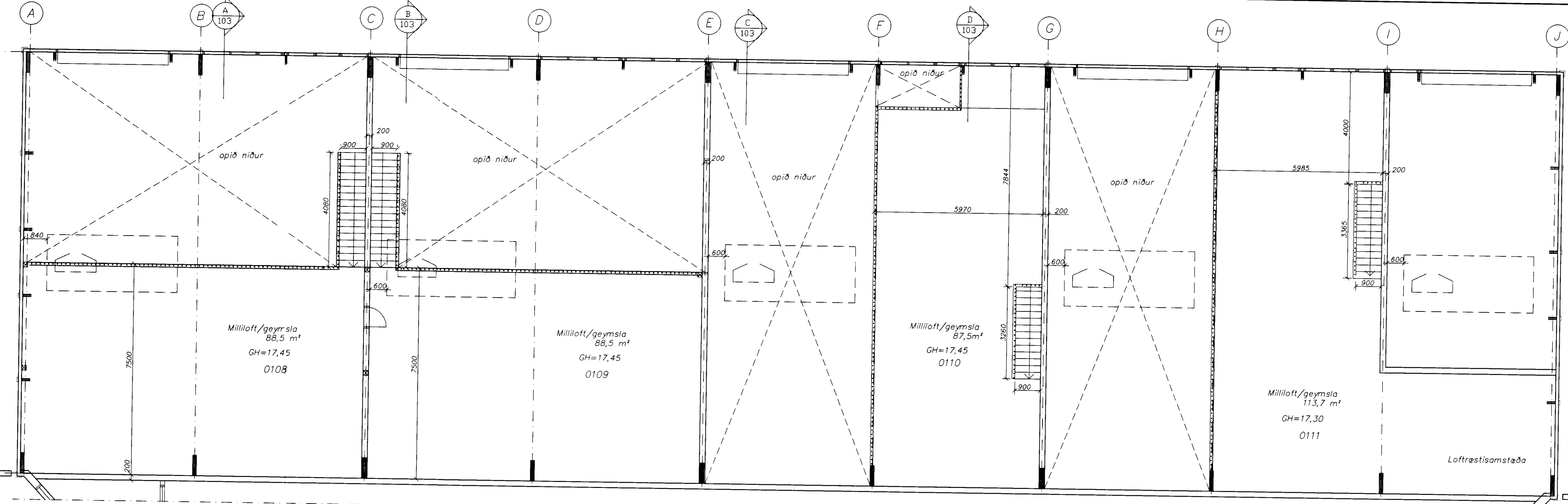
Grunnmynd-milliloft
