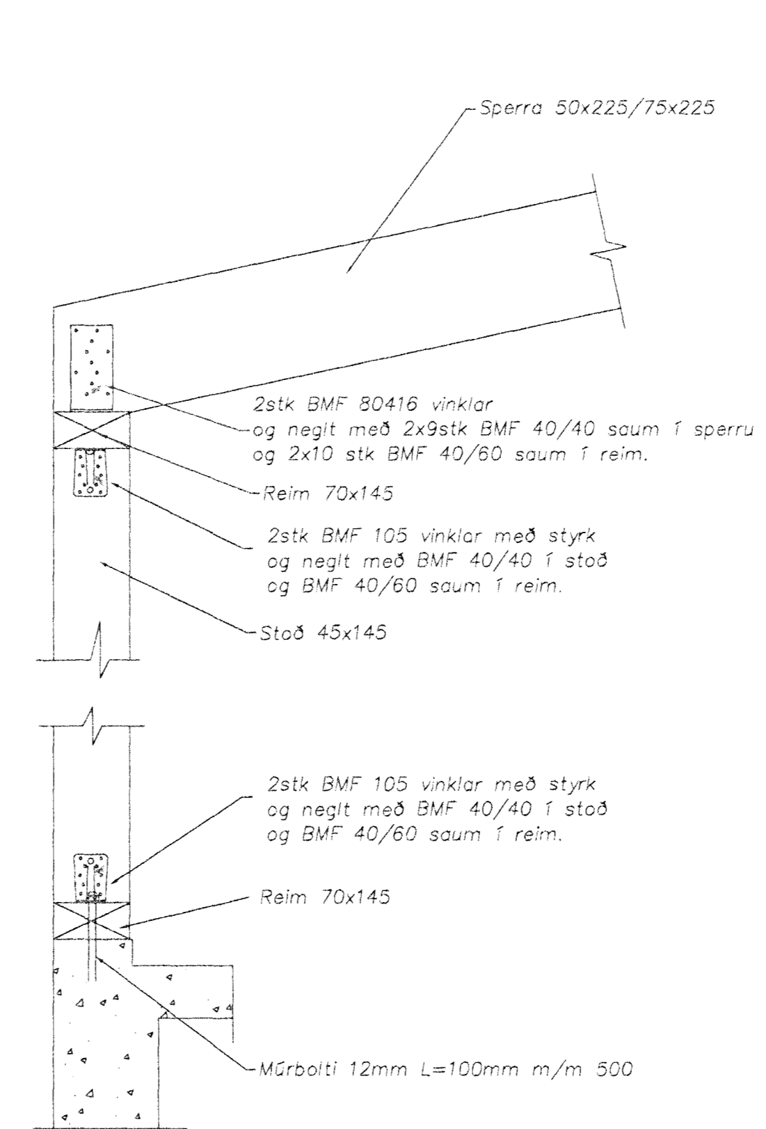
A Þakvirki sérteikningar Málsvæði 1:10
