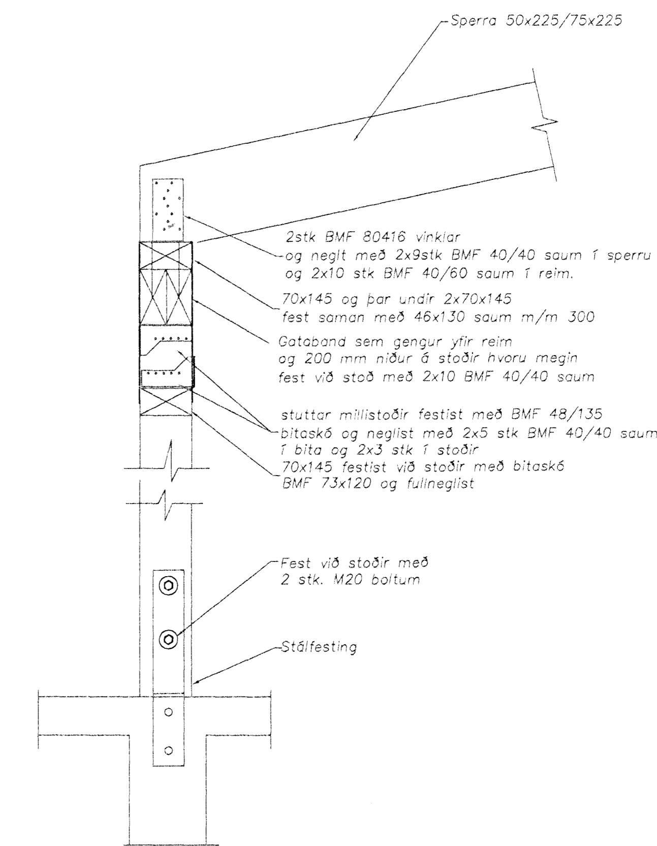
B Þakvirki sérteikningar Málsvæði 1:10
