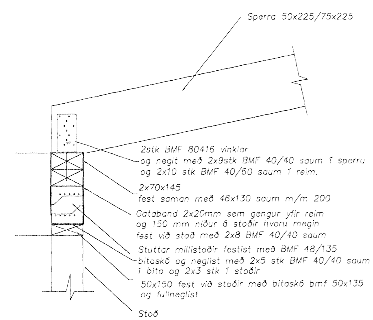
C Þakvirki sérteikningar Málsvæði 1:10
