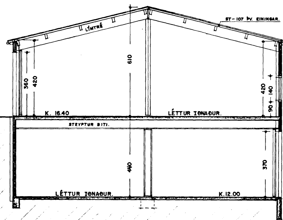
SNEIÐING. A - A 1:100
