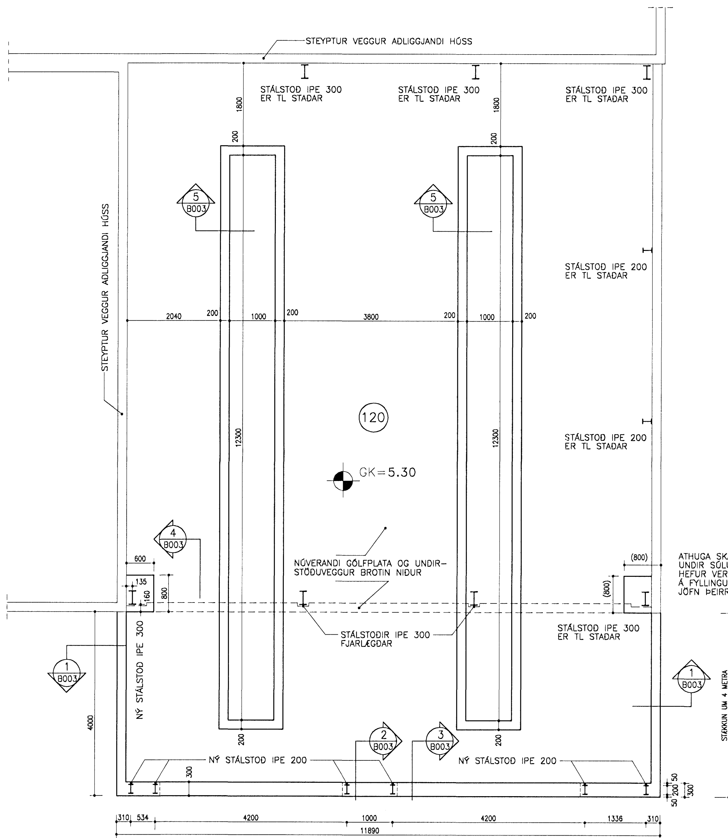
GRUNNMYND UNDIRSTÖÐUR 1:50
