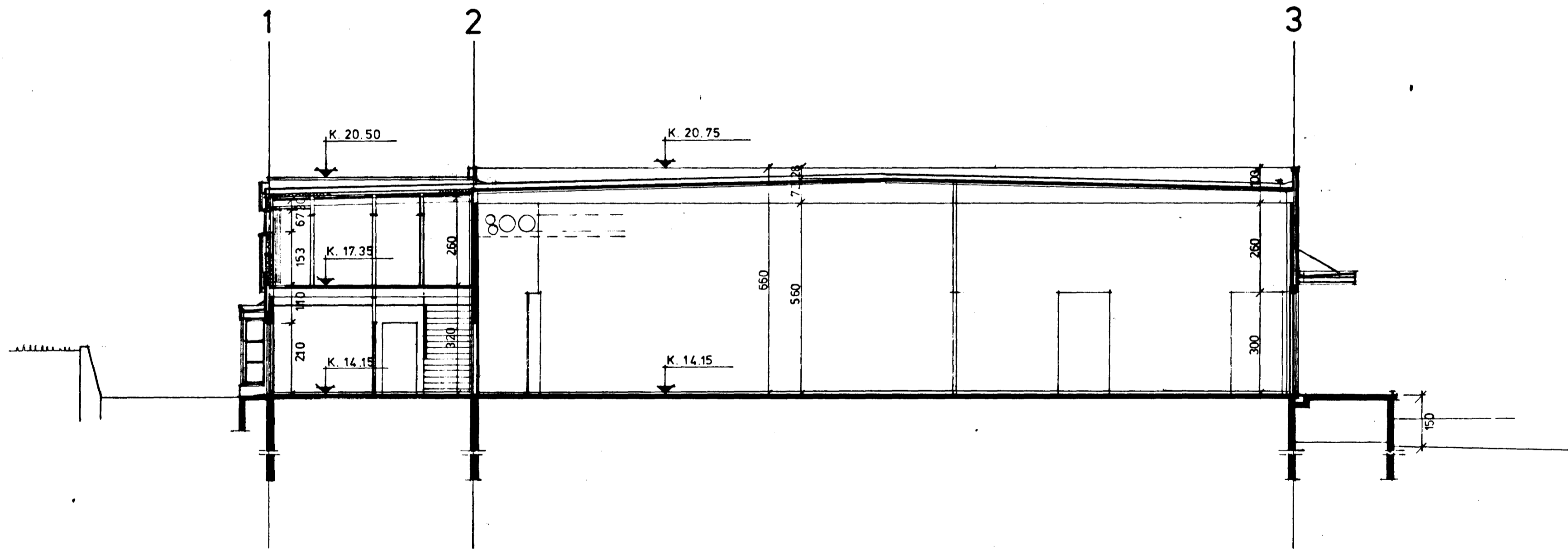
SNIÐ B-B
