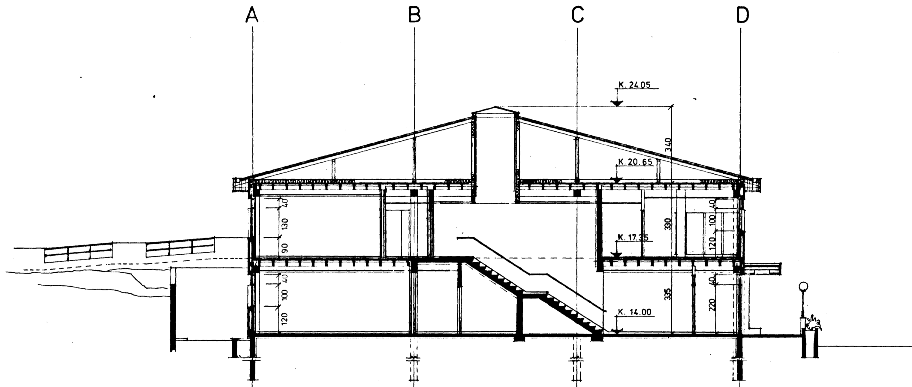
SNID A-A
