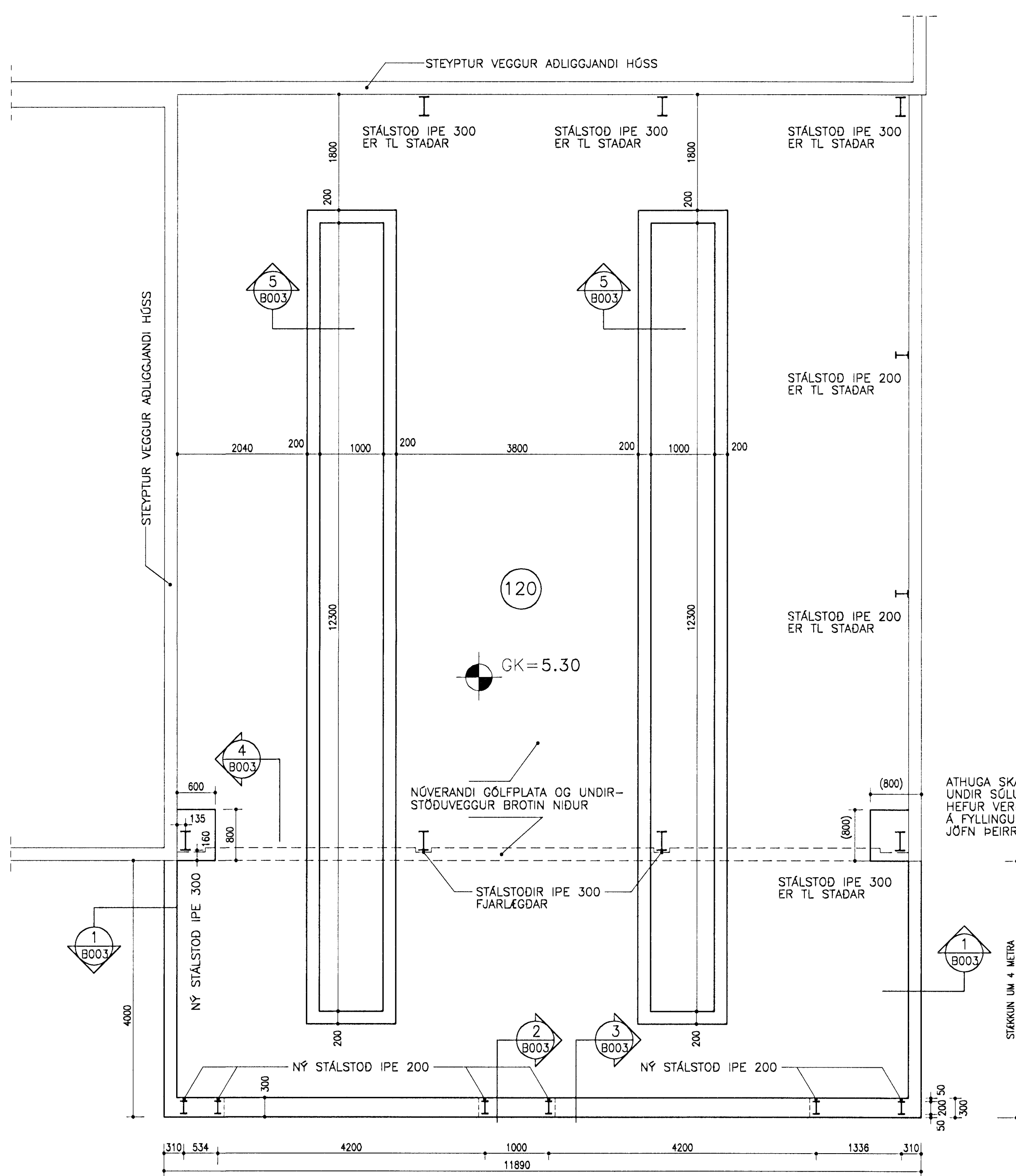
GRUNNMYND UNDIRSTÖÐUR 1:50
