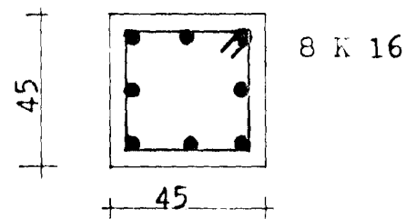
SÚGA S-1 1:20
