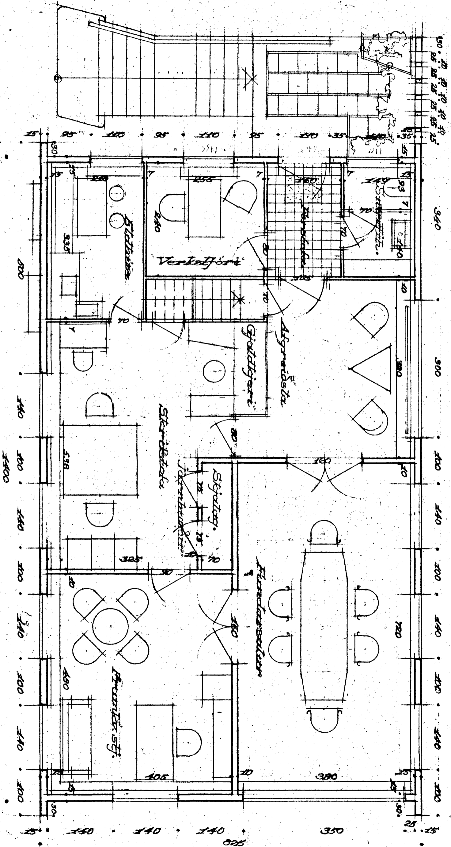
Grundmynd 1. hæðar
