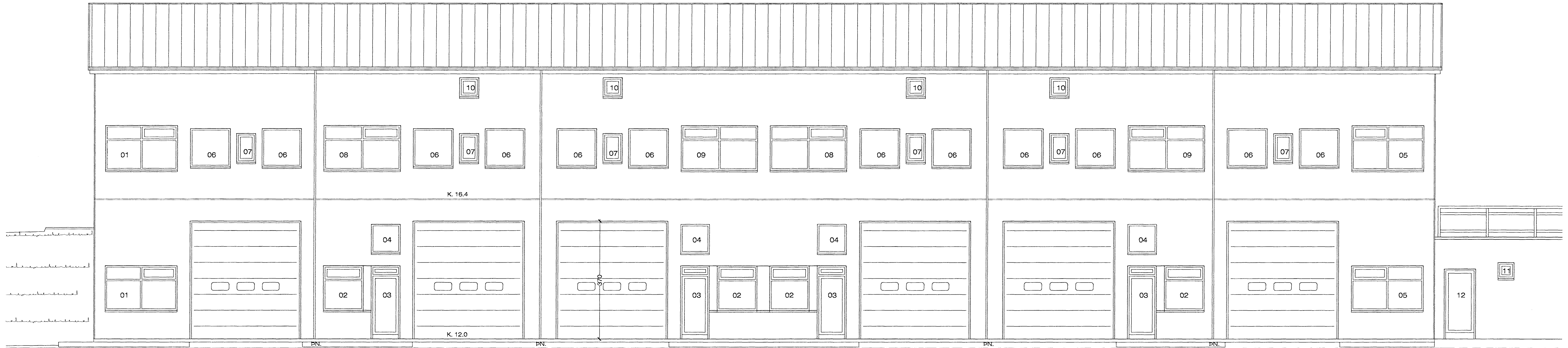
NORÐVESTURHLID M 1 : 50
