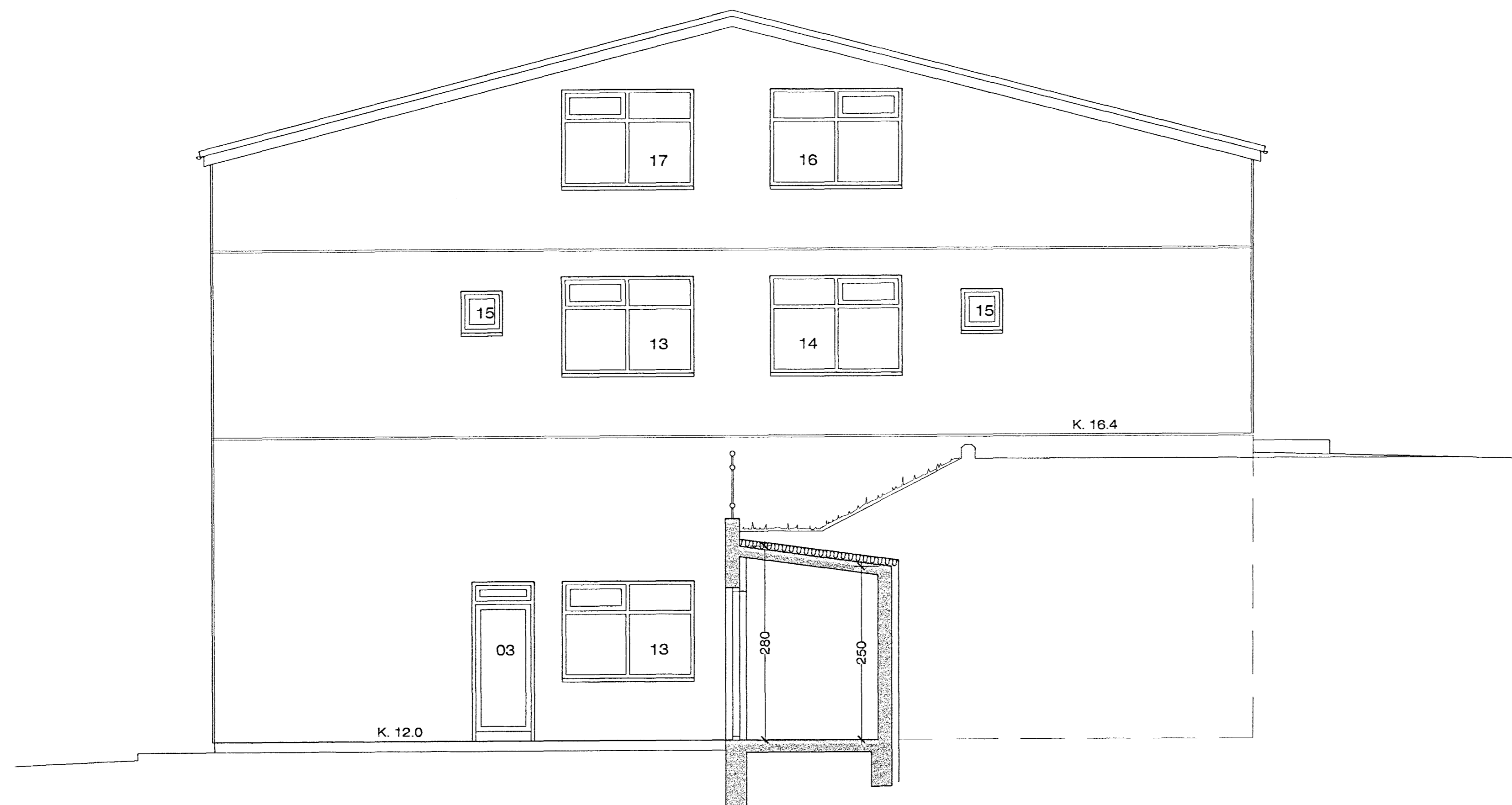
SUÐVESTURHLIÐ M 1 : 50
