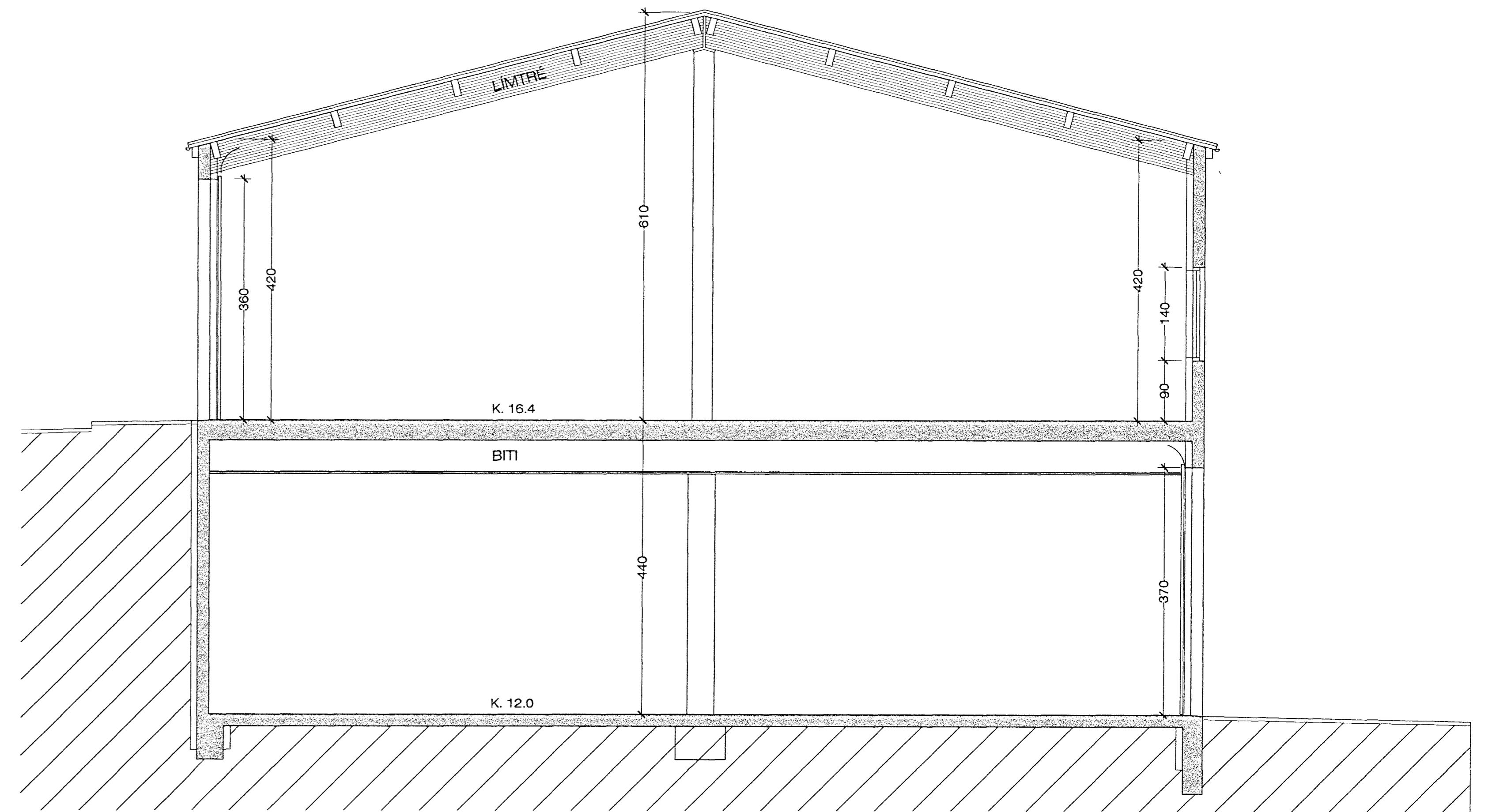
SNEIDING A - A M 1 : 50
