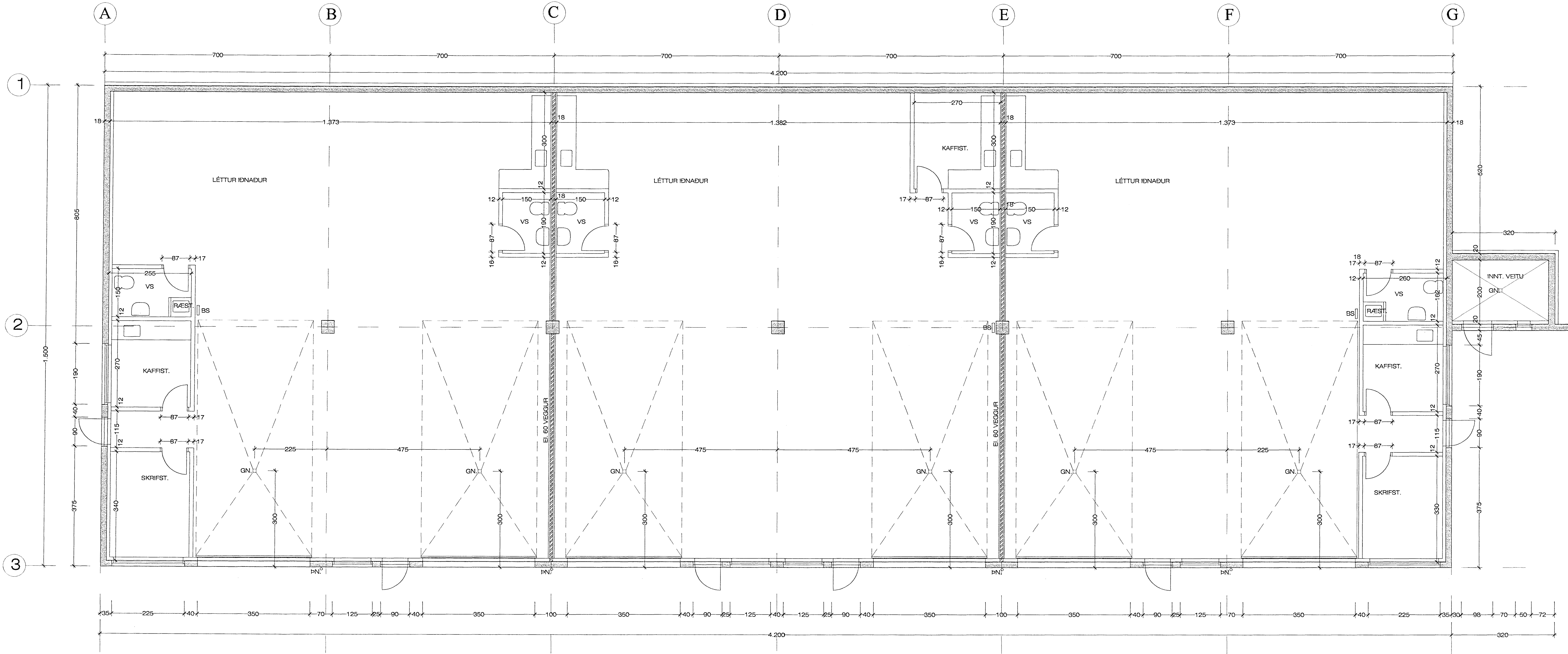
GRUNNMYND 1. HÆÐ M 1 : 50
