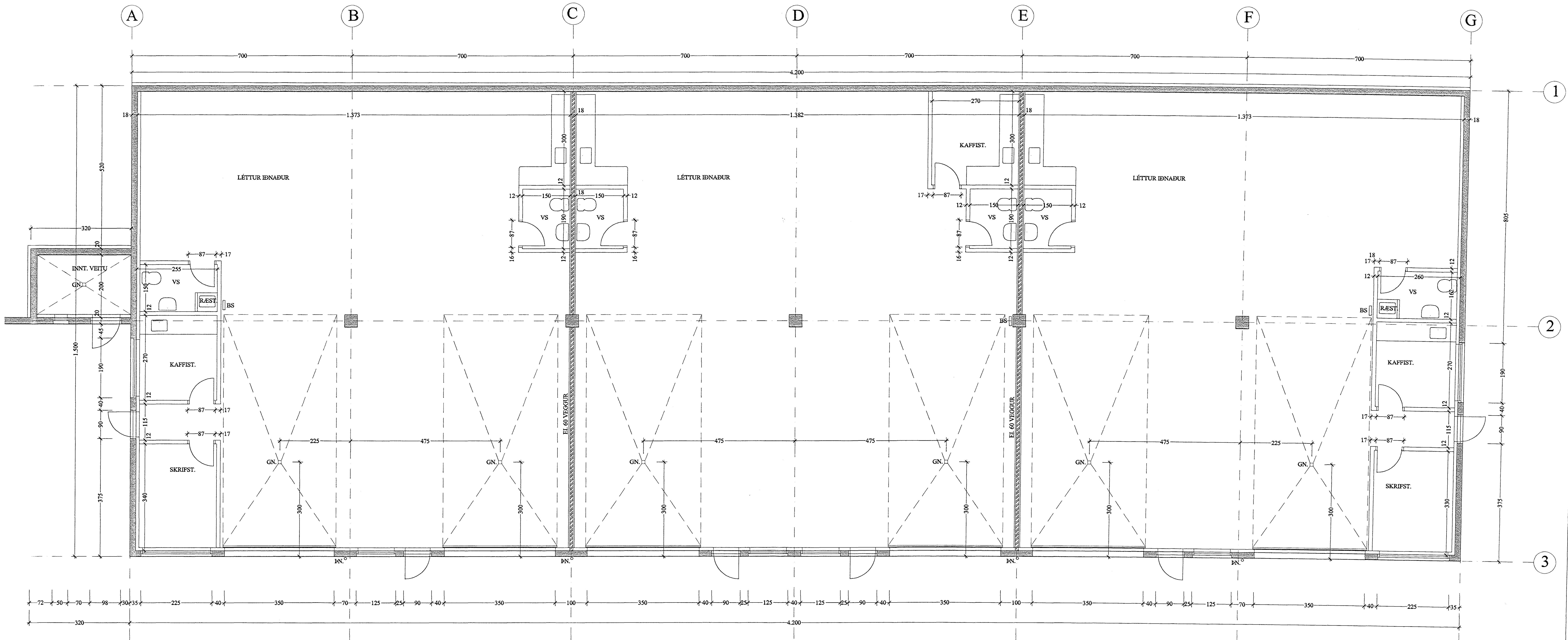
GRUNNMYND 1. HÆÐ M 1 : 50
