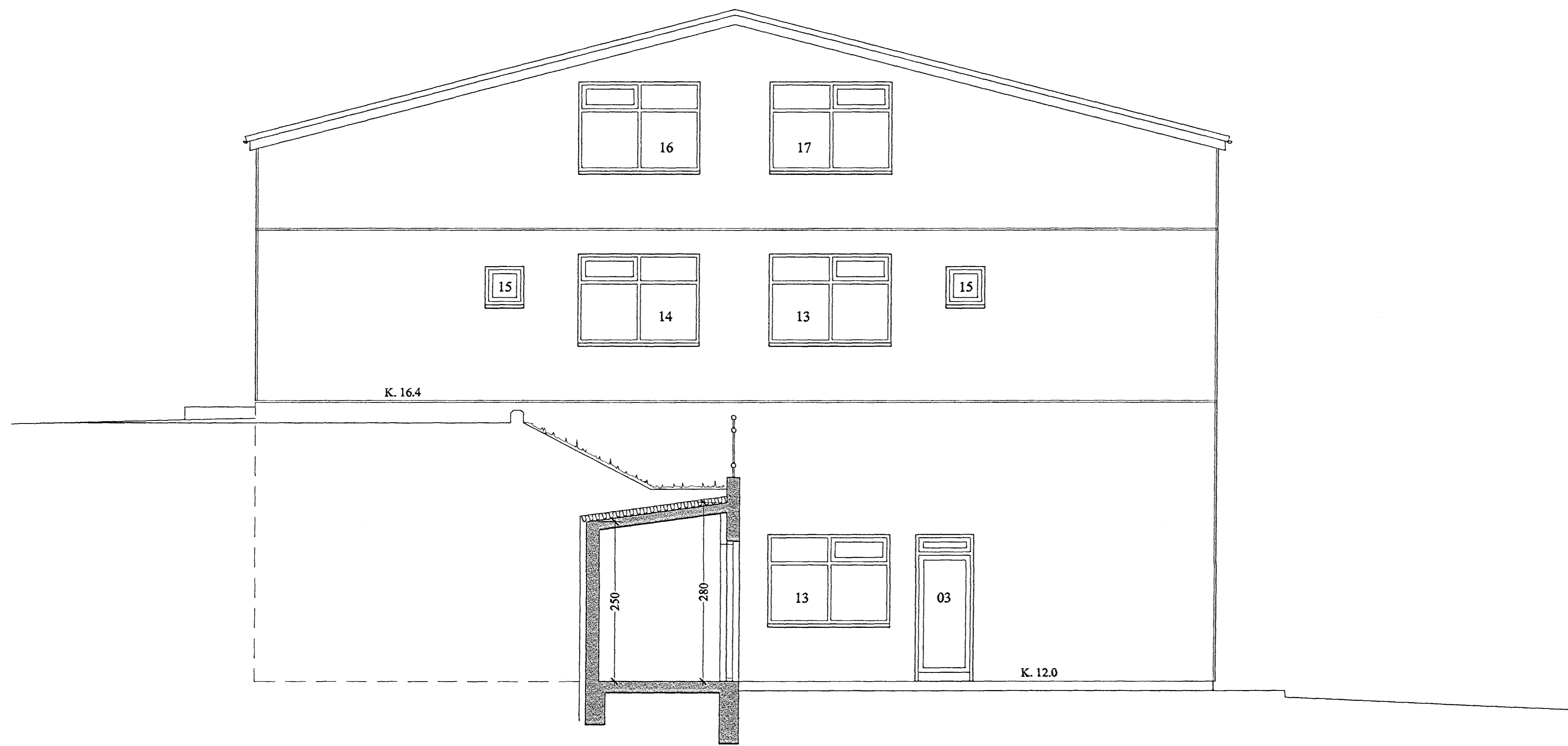
NORÐAUSTURHLIÐ M 1 : 50
