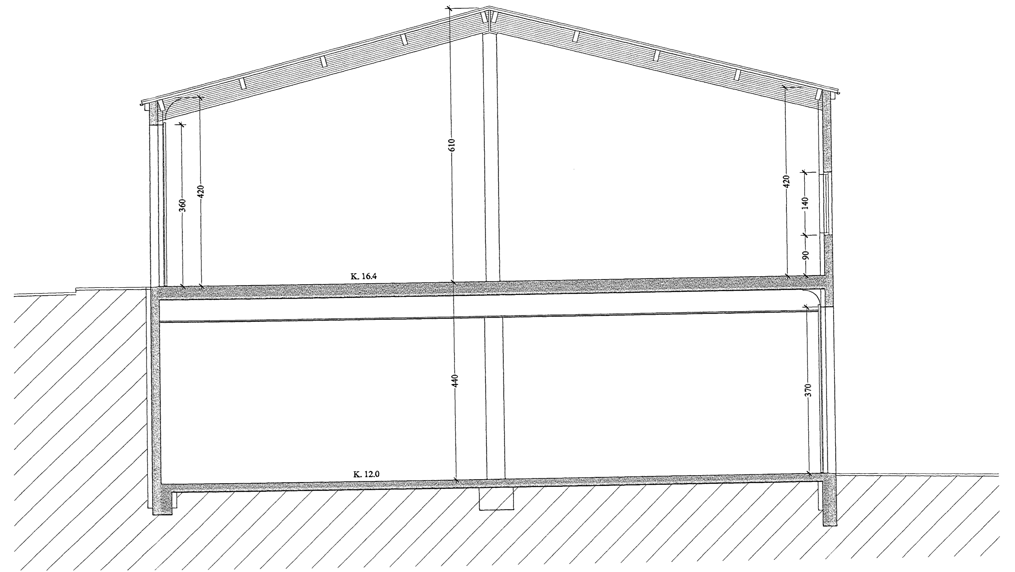
SNEIÐING A - A M 1 : 50
