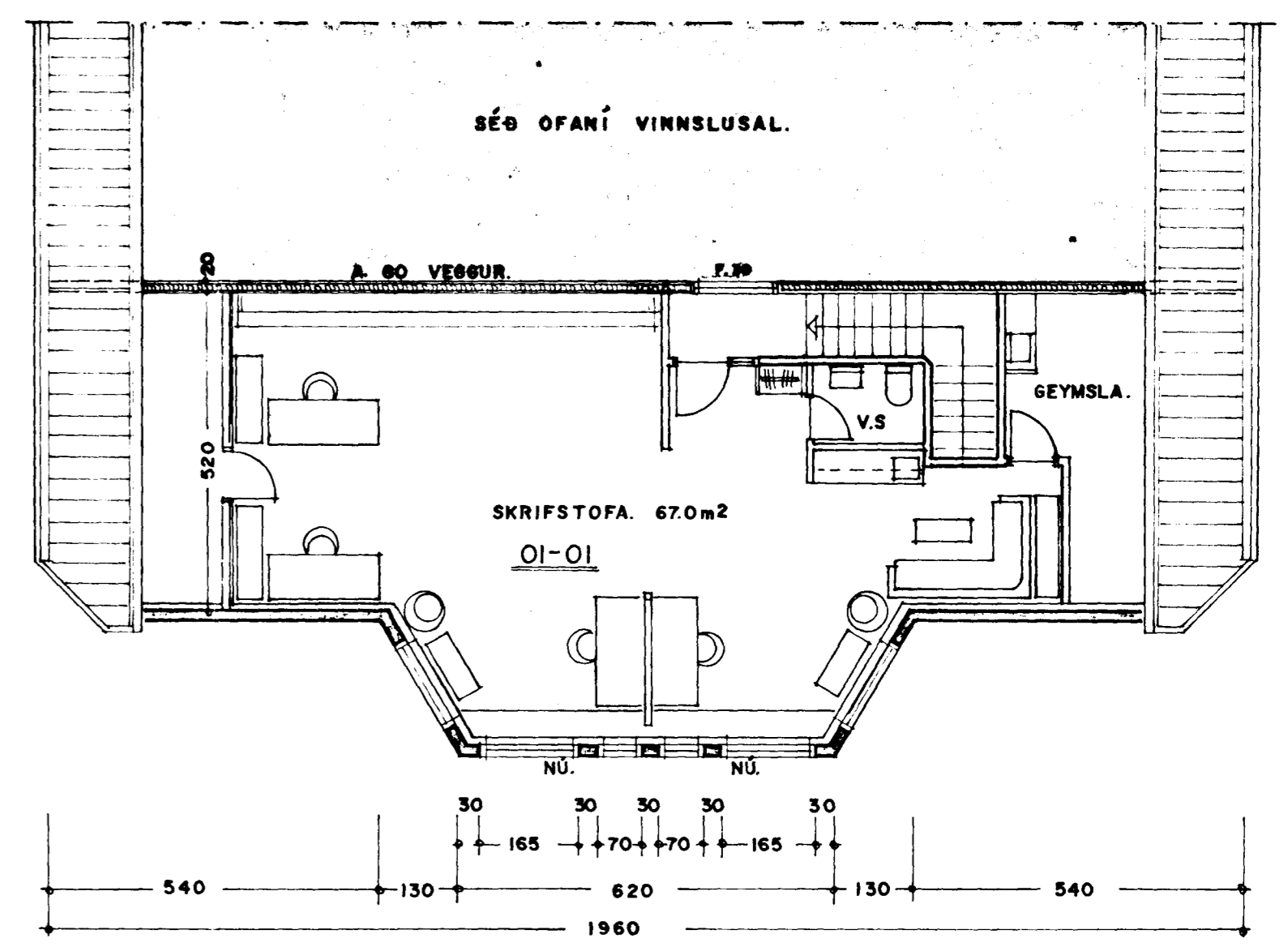
GRUNNMYND 2. HÆÐ MILLILOFT. 104.5 m 2
