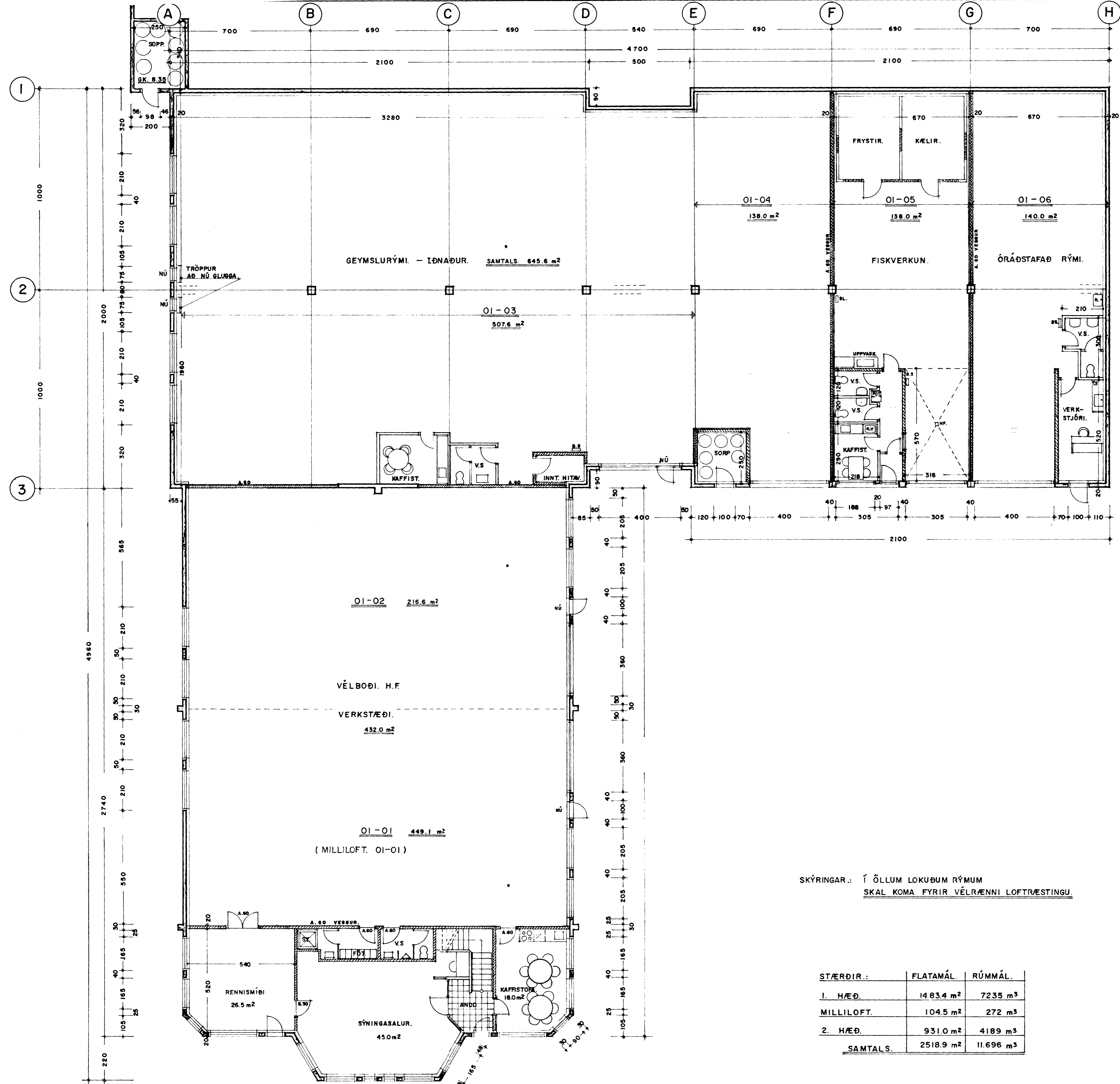
GRUNNMYND 1. HÆÐ 1483.4 m 2
