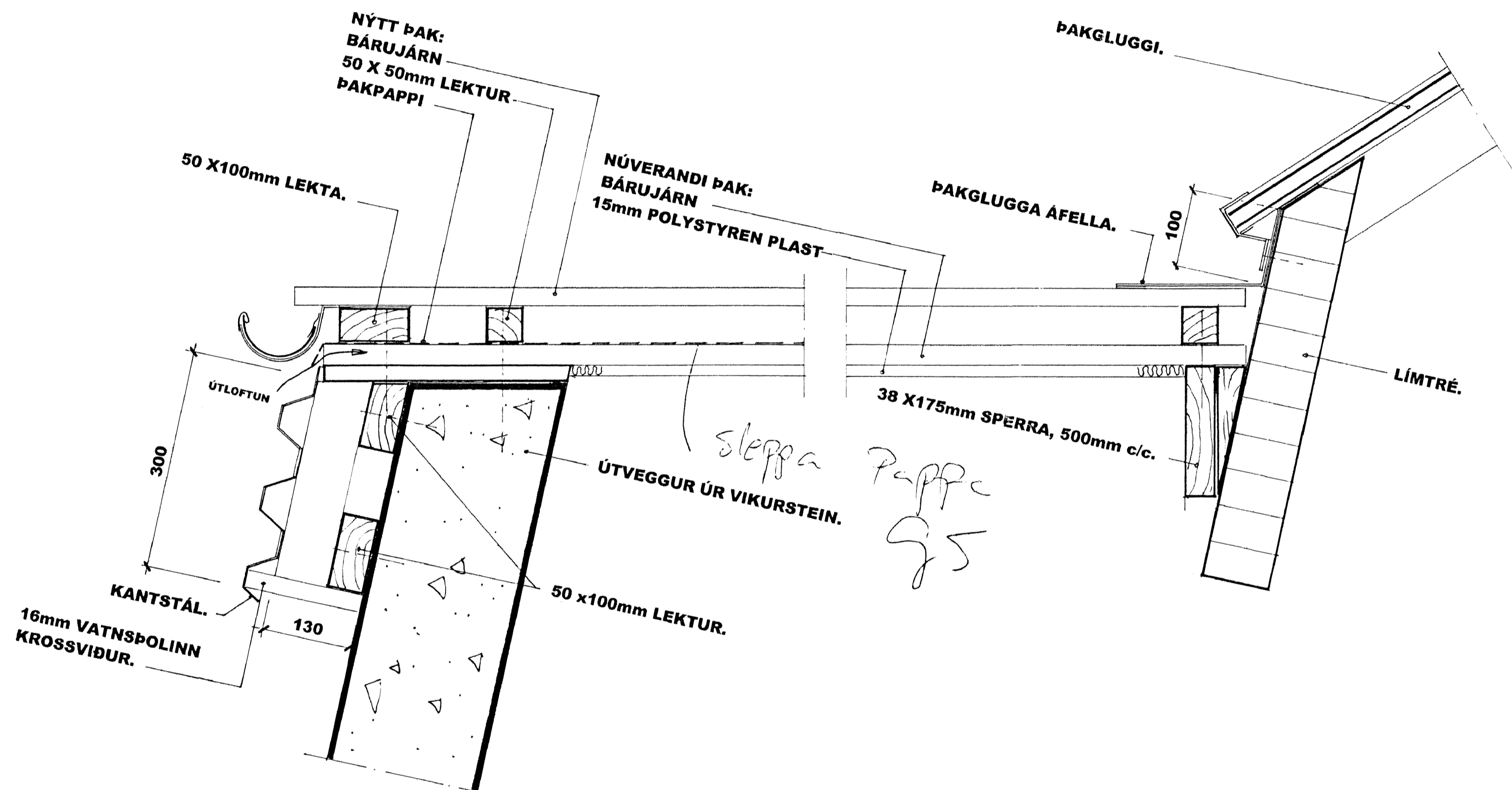
FRÁGANGUR ÞAKS VIÐ RENUU OG ÞAKGLUGGA
