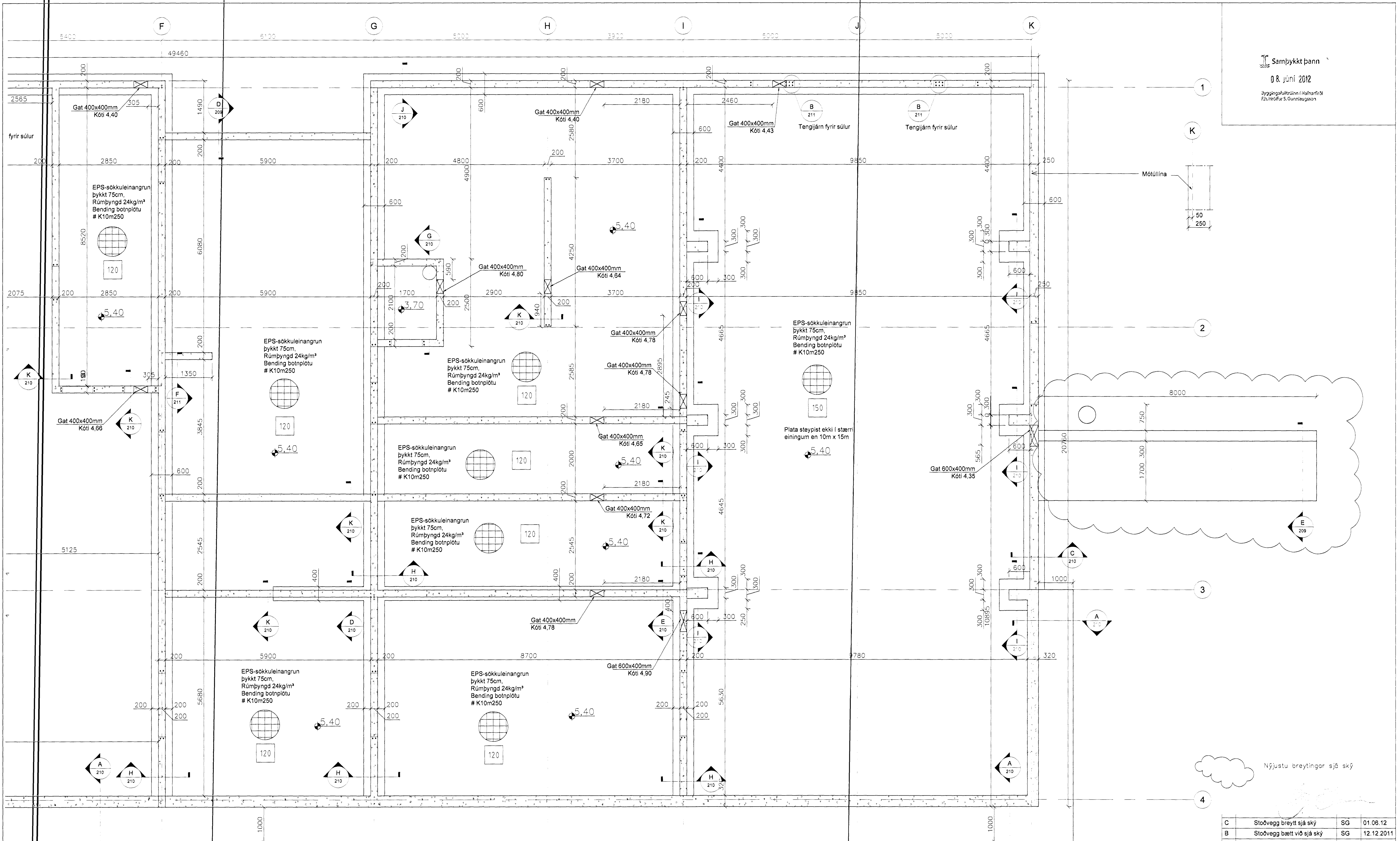
Grunnmynd undirstöður = 50 mm
