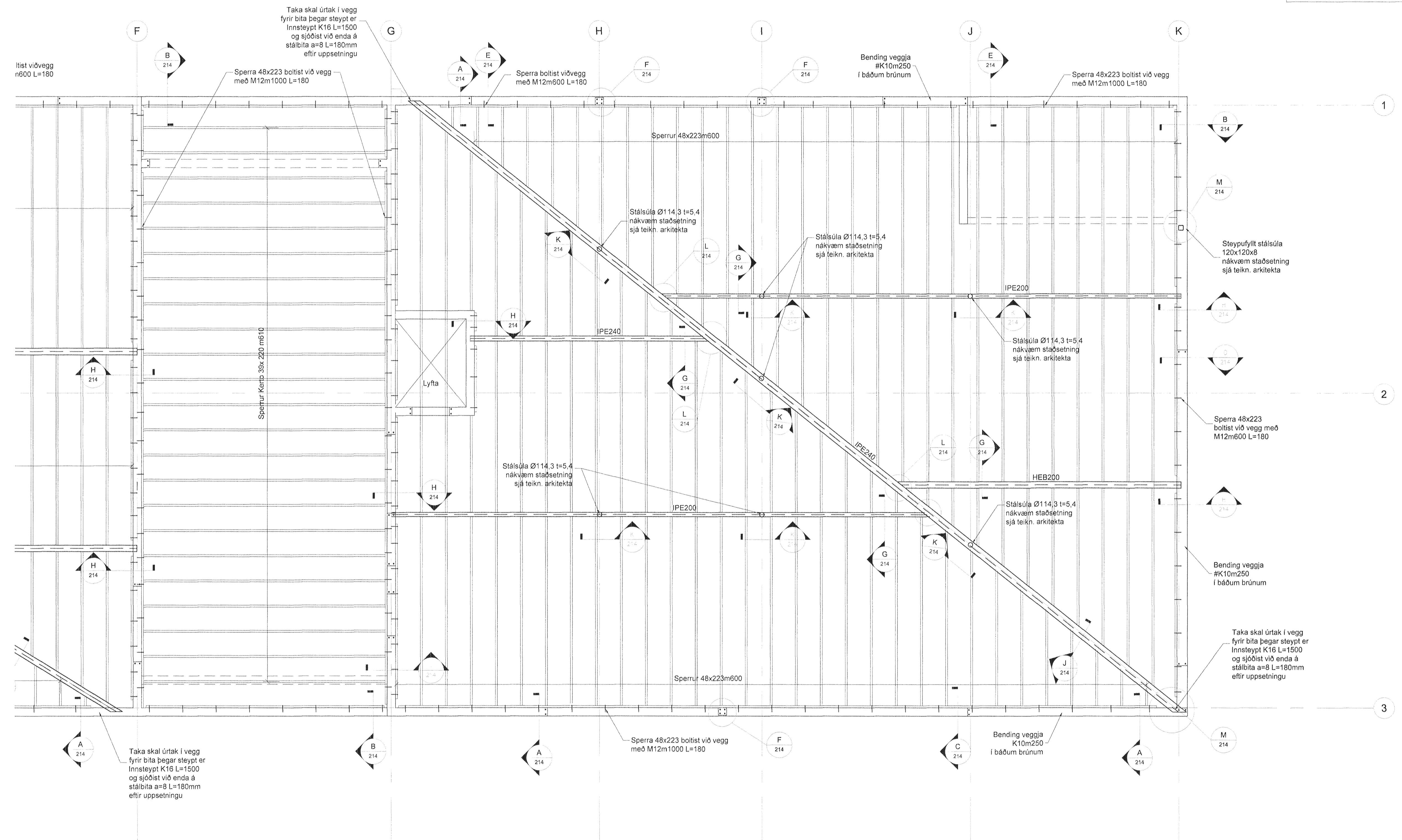
Grunnmynd þaks 1 = 50 mm
