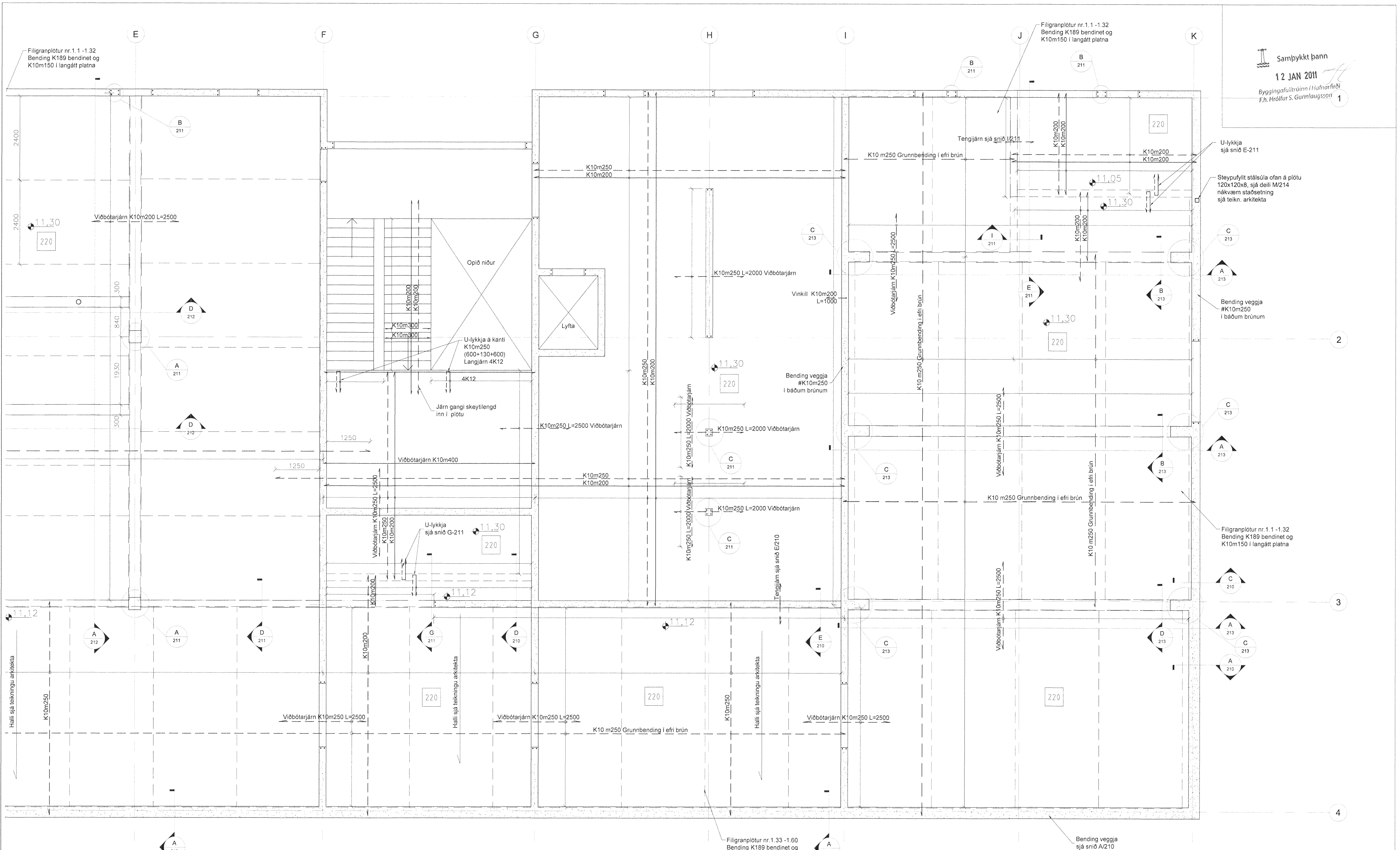
Grunnmynd plata 2. hæð 1 = 50 mm
