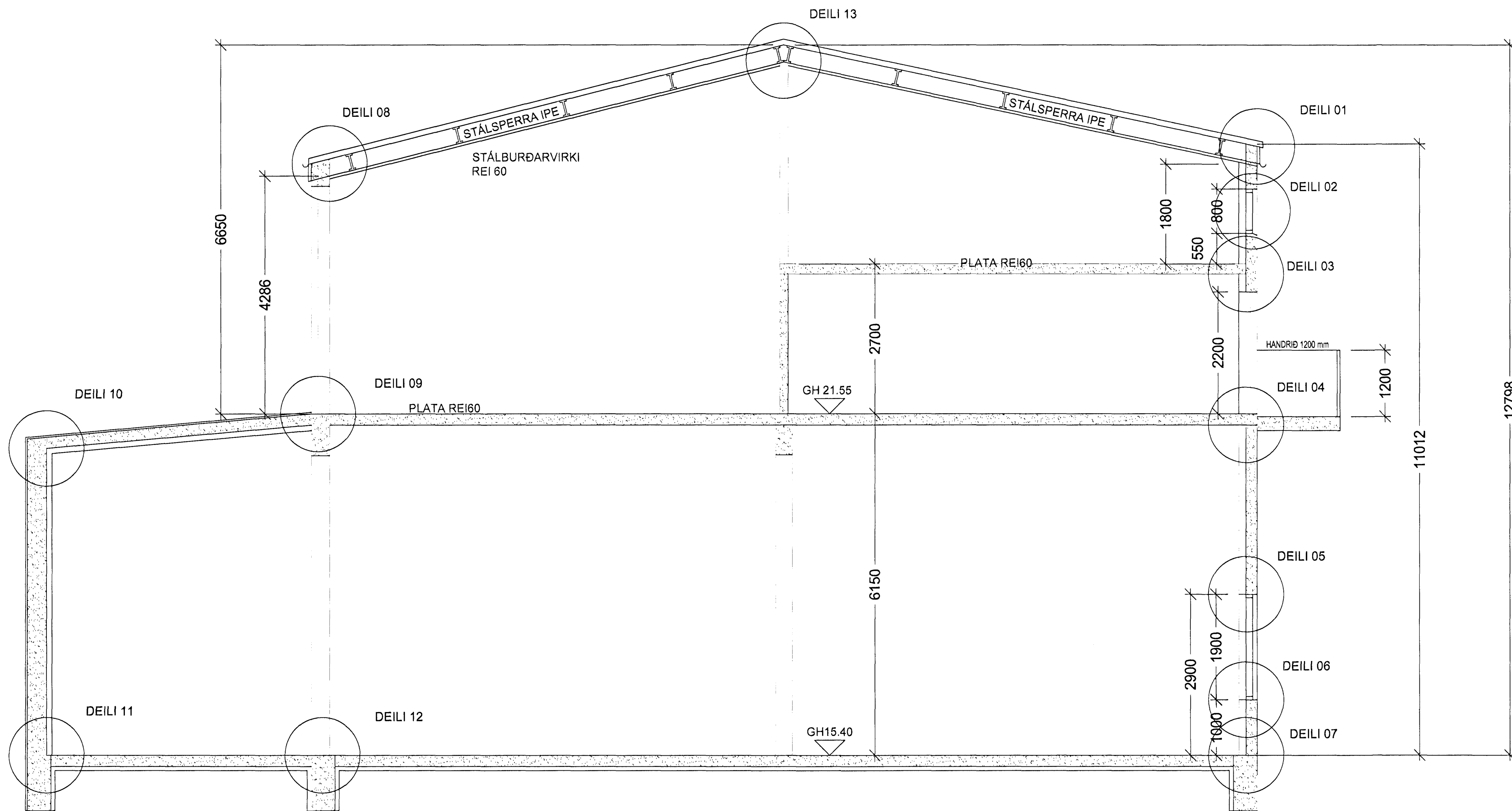
SNID A-A 1:50
